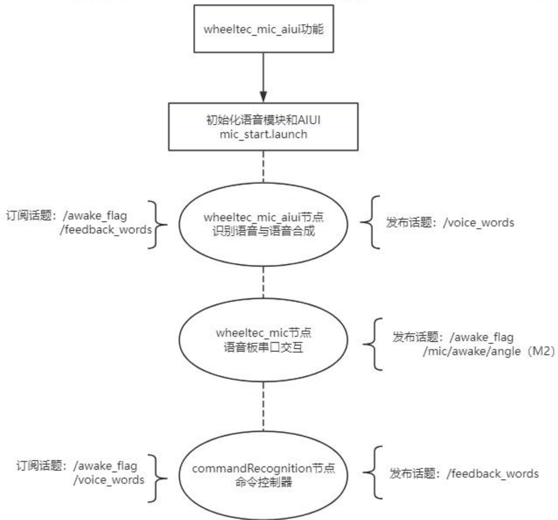
图 4-1 AIUI 功能节点示意图
