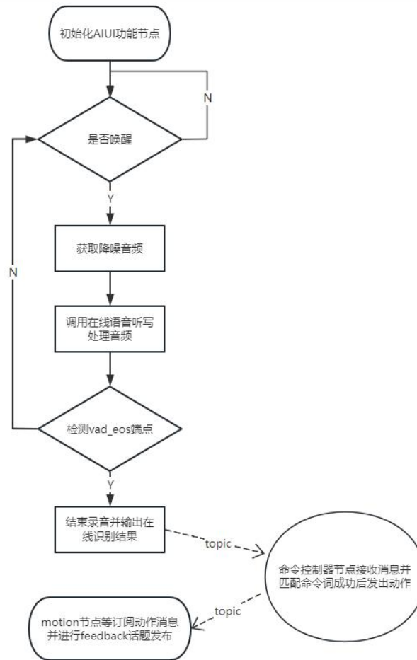
图 4-3 主要 AIUI 交互功能流程图
