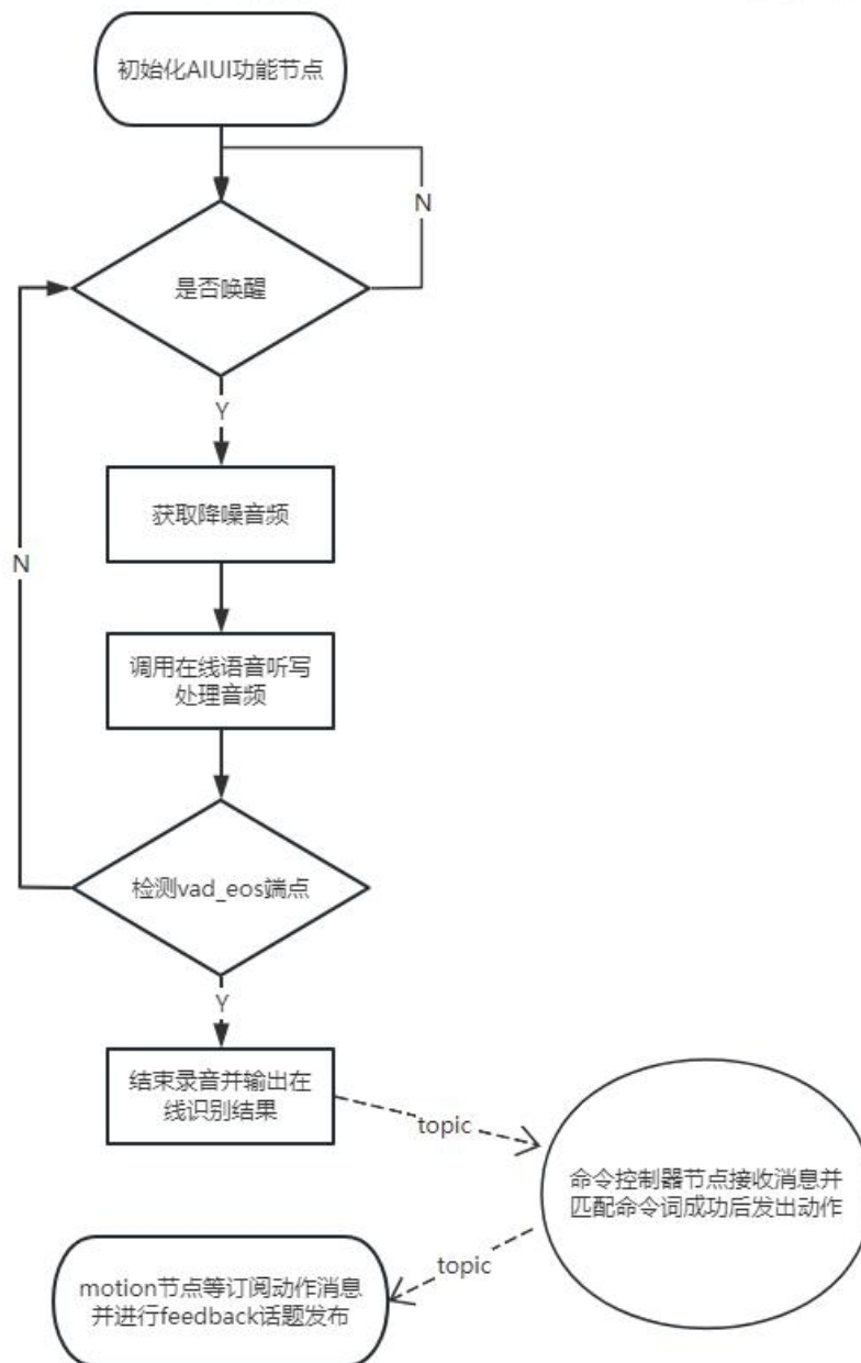
图 4-3 主要 AIUI 交互功能流程图
