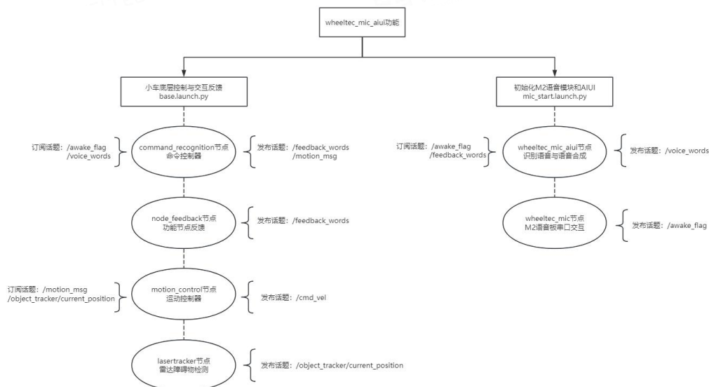
图 4-1 AIUI 功能 ROS2 节点示意图
