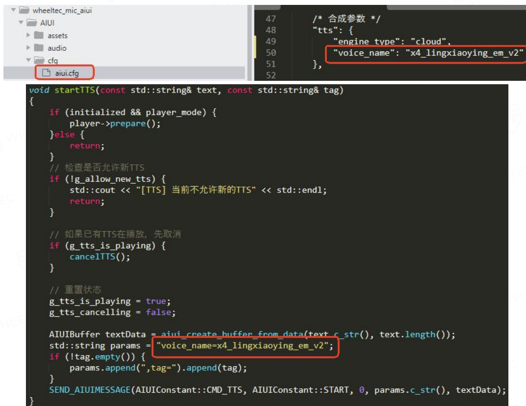
图 3-4-5 语音合成发音人名称设置
