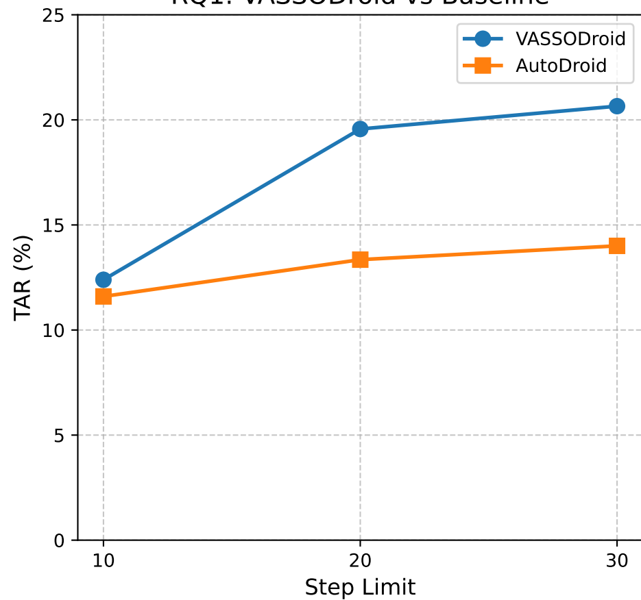
RQ1: VASSODroid vs Baseline
