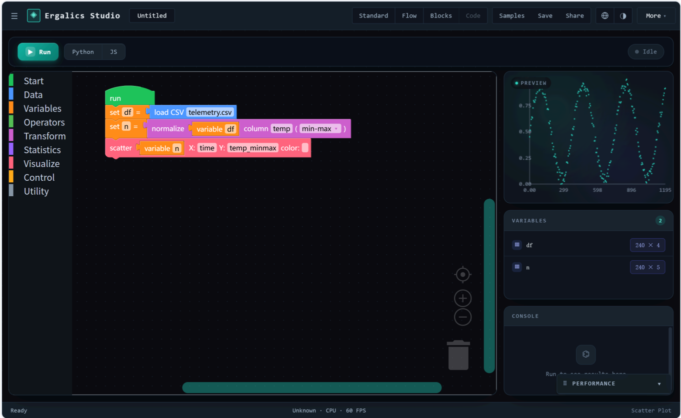
积木模式：类 Scratch 画布，绿色"运行时"帽子区块是脚本唯一入口，积木图编译为共享 IR 由内置解释器逐节点执行。
