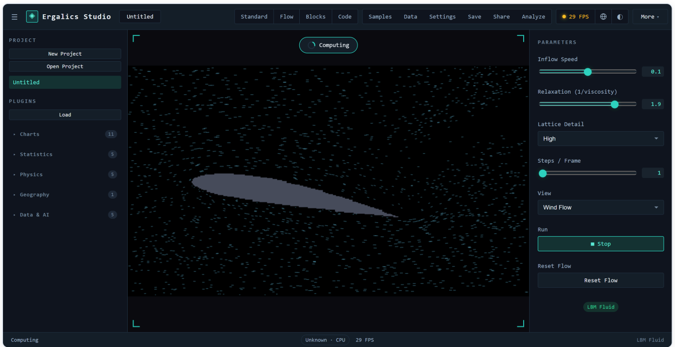
格子 Boltzmann 流体：D2Q9 通道流绕翼型障碍物，展示卡门涡街与机翼绕流，GPU 三内核逐步计算 + CPU 降级。
