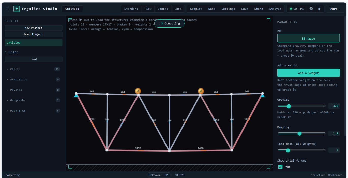
结构力学：铰接桁架实时承重，杆件按轴力着色，超载时依次断裂直至整体垮塌。
