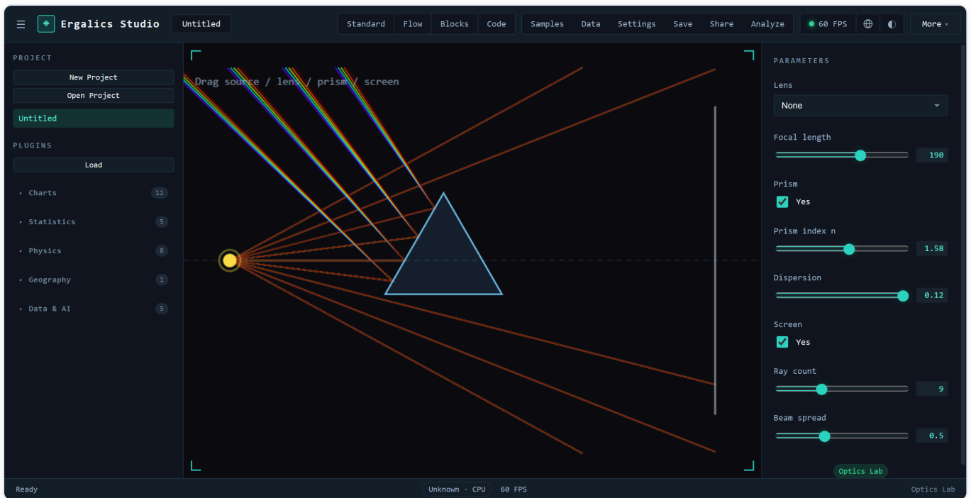
光学实验：几何光学光线追踪，白光束经三棱镜折射色散，薄透镜成像焦距演示，元件均可拖动。
