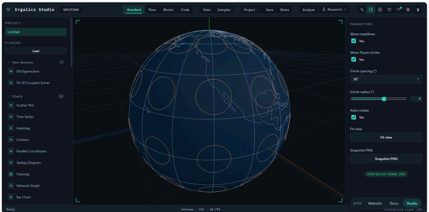
交互地球仪（3D）：可拖拽旋转、滚轮缩放的真三维地球仪，Natural Earth 110m 海岸线贴于球面，叠加球面 Tissot 变形圆并支持自动自转。
