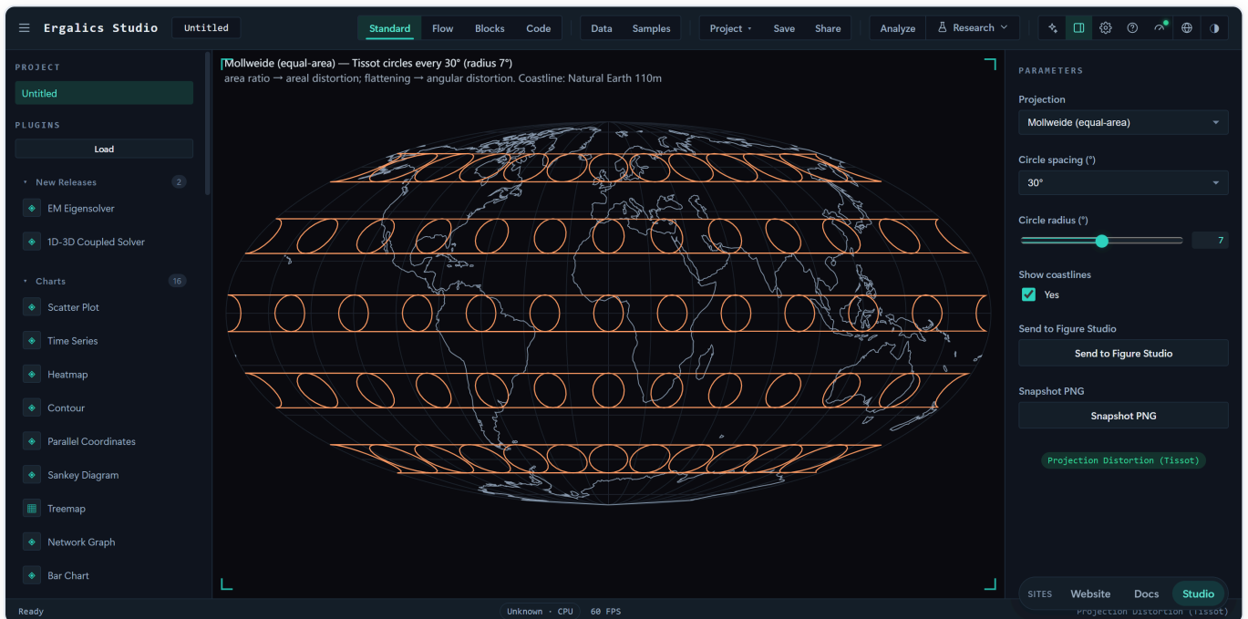
投影变形（Tissot 圆）：在七种投影下绘制世界海岸线与 Tissot 变形圆，圆面积比表征面积变形、扁率表征角度（形状）变形；图中为保持等积性质的 Mollweide 投影。
