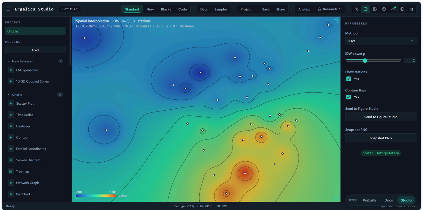
空间插值：将离散站点观测值网格化——图中 IDW ( p=2 ) 对 31 站点生成热力面与等值线，附 LOOCV 交叉验证 RMSE / MAE 与 Moran's I 空间自相关检验。
