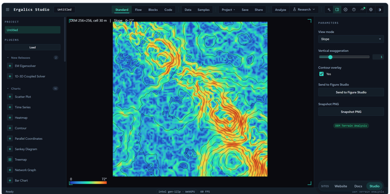
DEM 地形分析 (坡度视图)：按 Horn 法计算坡度 (0-72°) 并叠加等高线，另一模式给出山体阴影，用于提取地形坡度与坡向。
