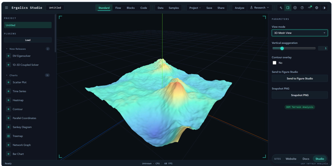
DEM 地形分析 (3D Mesh 视图)：解析 ESRI ASCII Grid 高程数据，三维曲面按高程设色、垂直夸张系数可调，并可叠加等高线。
