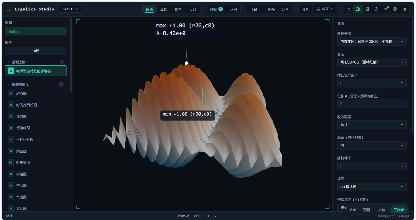
3D 模式场: cavity_small 配合块 LOBPCG 内核, 展示 \lambda = 8.42\text{e}+0 的模式
