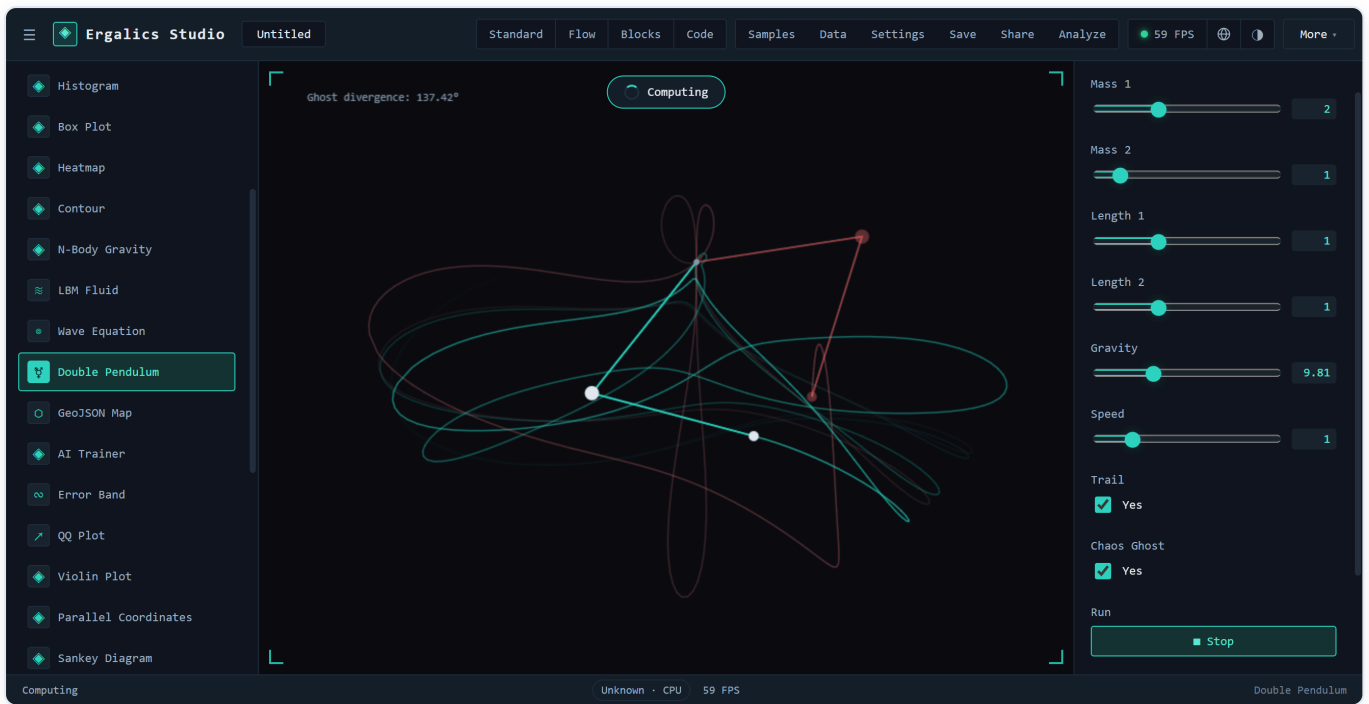
双摆：RK4 积分，主摆与初始角仅差 0.001 rad 的"幽灵摆"并行演化，轨迹快速发散，直观展示混沌对初值的敏感依赖。
