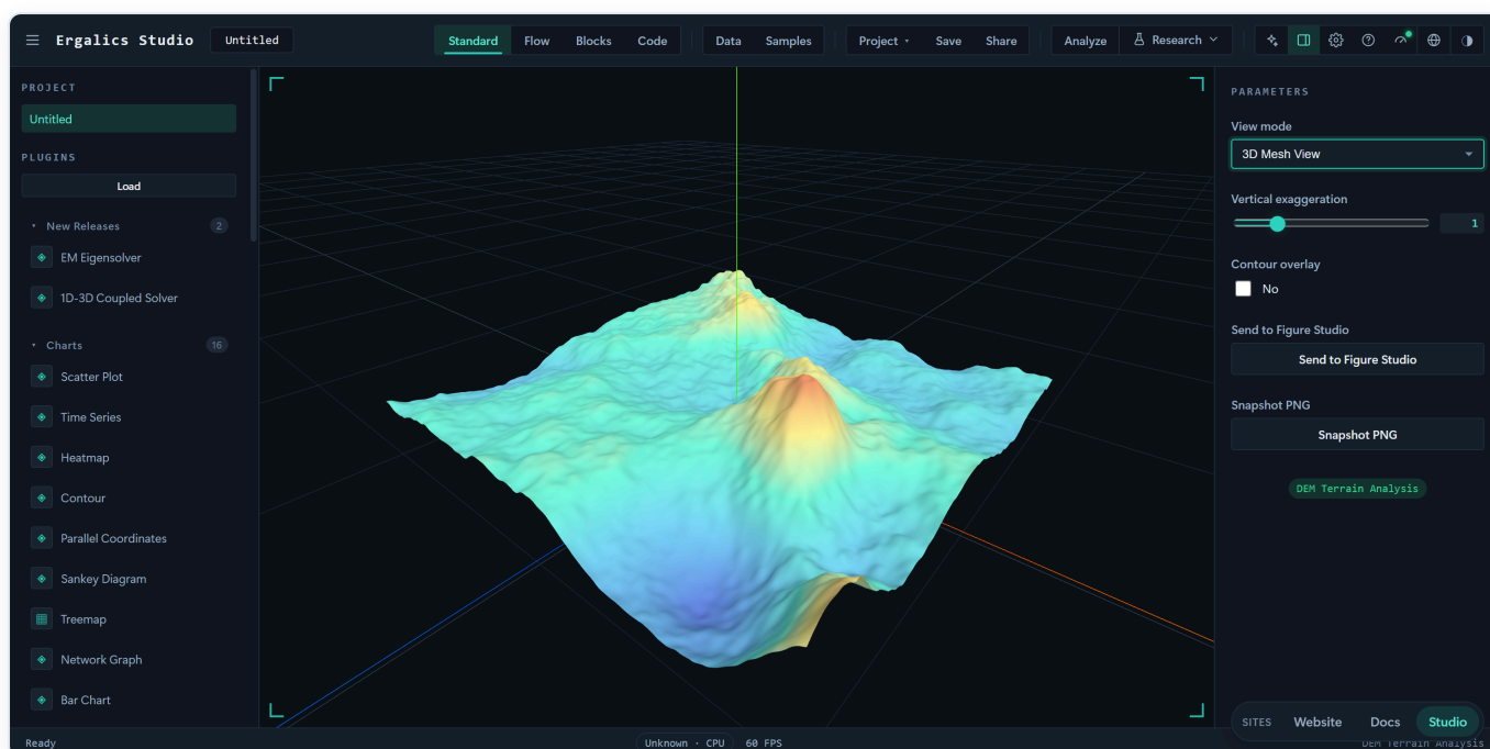
DEM 地形分析：解析 ESRI ASCII Grid 高程数据，三维曲面按高程设色、垂直夸张系数可调，并可叠加等高线。
