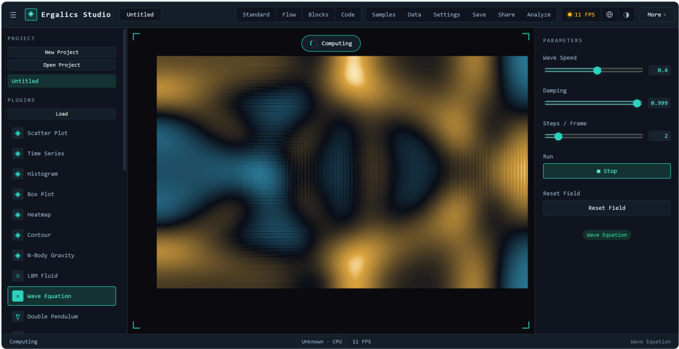
波动方程：二维有限差分模拟高斯脉冲 / 双源干涉 / 双缝衍射，leapfrog 内核逐步积分，图为双缝衍射干涉。
