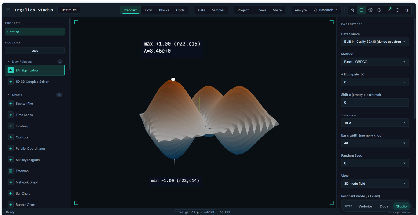
电磁谐振特征值求解器：Lanczos / LOBPCG / Jacobi-Davidson 求稀疏厄密特征对并做真实残差认证，图中为微波腔体 3D 模式场。
