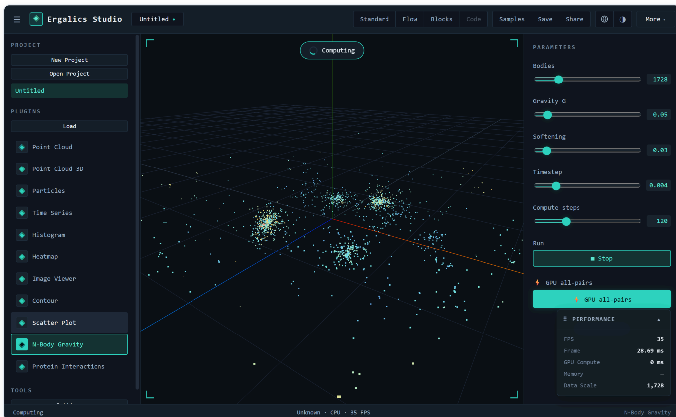
N-Body 引力
