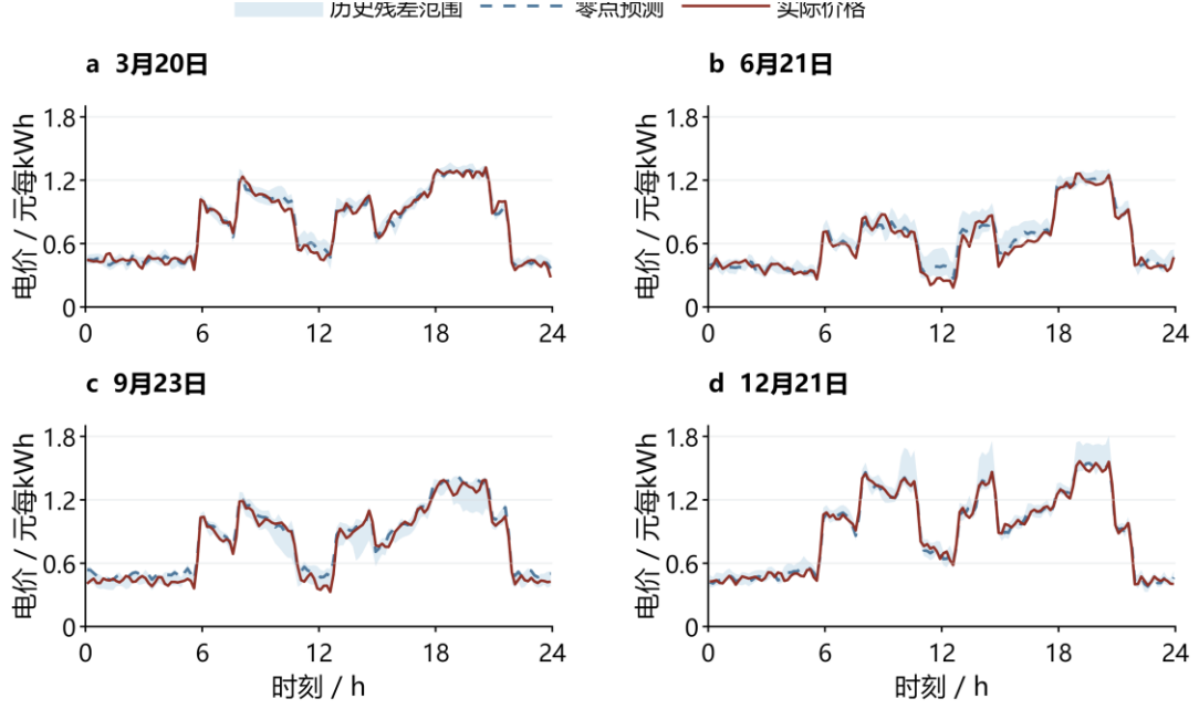
图 11 波动价格的预测偏差与历史残差范围
