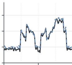
(c) 9月23日
