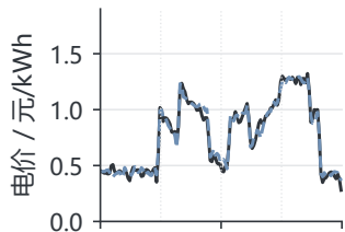
(a) 3月20日
