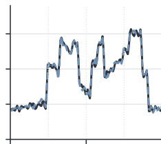
(d) 12月21日
