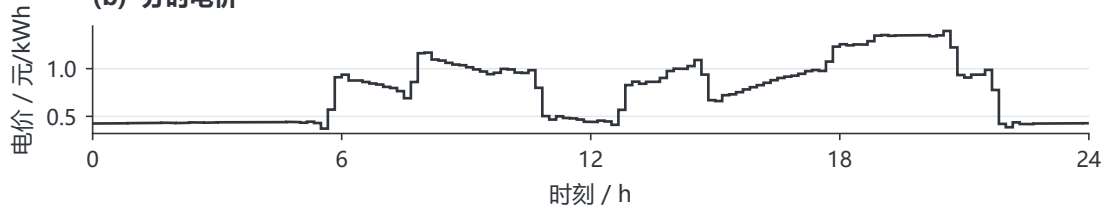
(b) 分时电价
