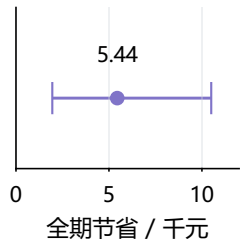
d 全期与95%区间
