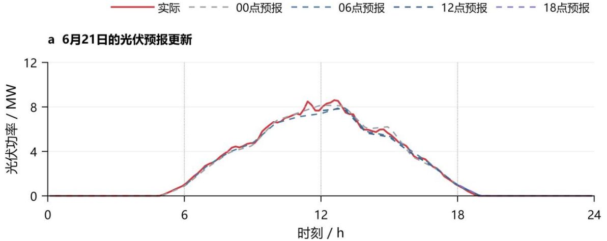
图 8 四个发布版本的光伏预报
