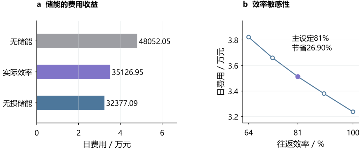
图 4 储能的净收益及效率对最优费用的影响
