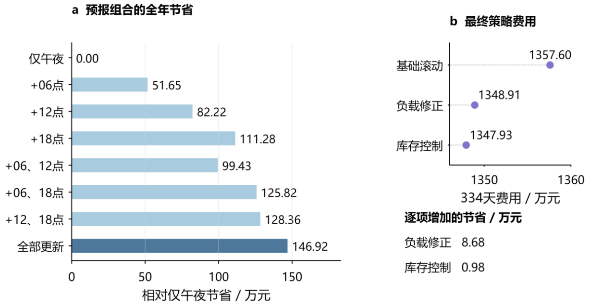
图 10 预报更新组合的全年收益与第三问最终费用
