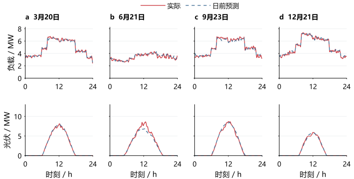
图 6 四个指定日期的负载与光伏日前预测
