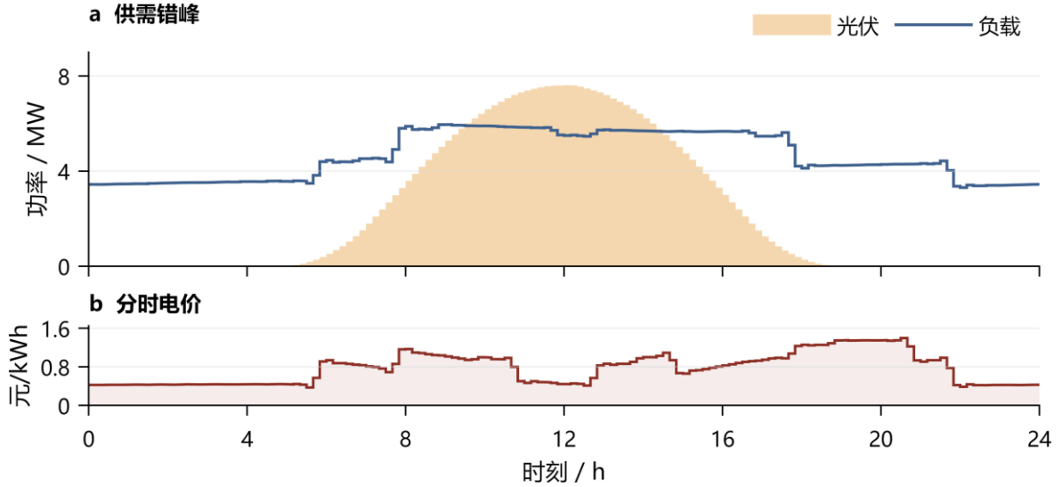
图 2 第一问供需曲线与分时电价
