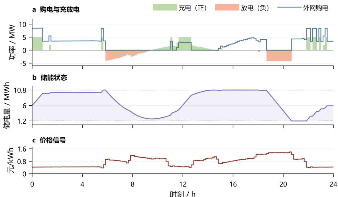
图 3 第一问电价驱动的购电与储能运行
