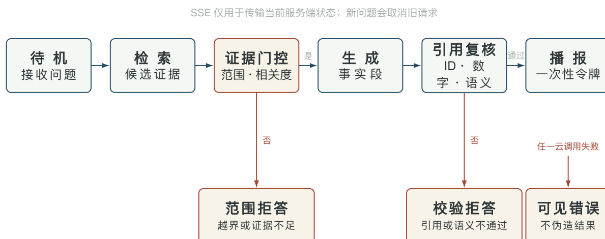
图 5: 查询、拒答、错误与播报的前后端状态机
