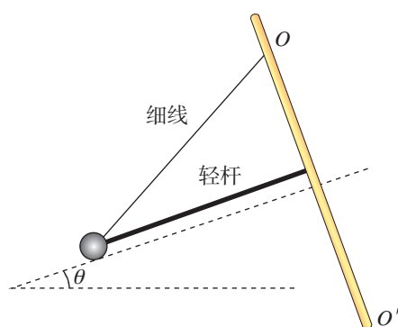
图研-3 杆线摆
