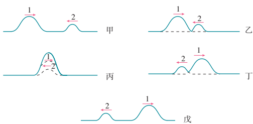
图 3.4-1 波的叠加
