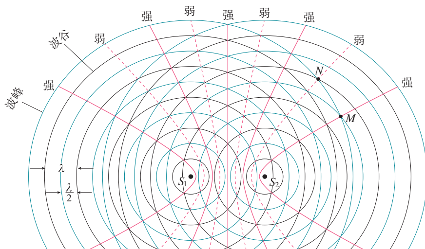
图 3.4-3 波的干涉示意图
