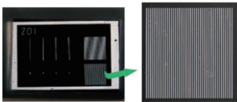
图 4.5-5 透射光栅
