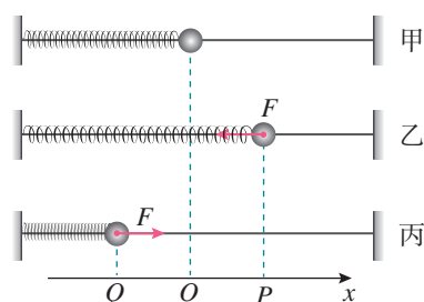
图 2.3-1 简谐运动的回复力
