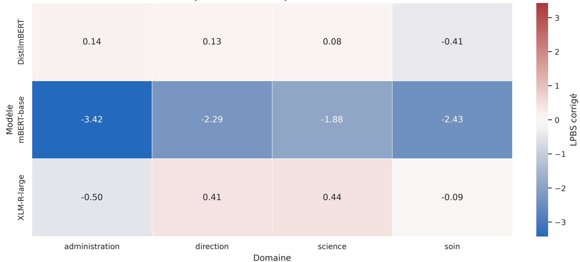
LPBS par domaine et par taille de MLM
