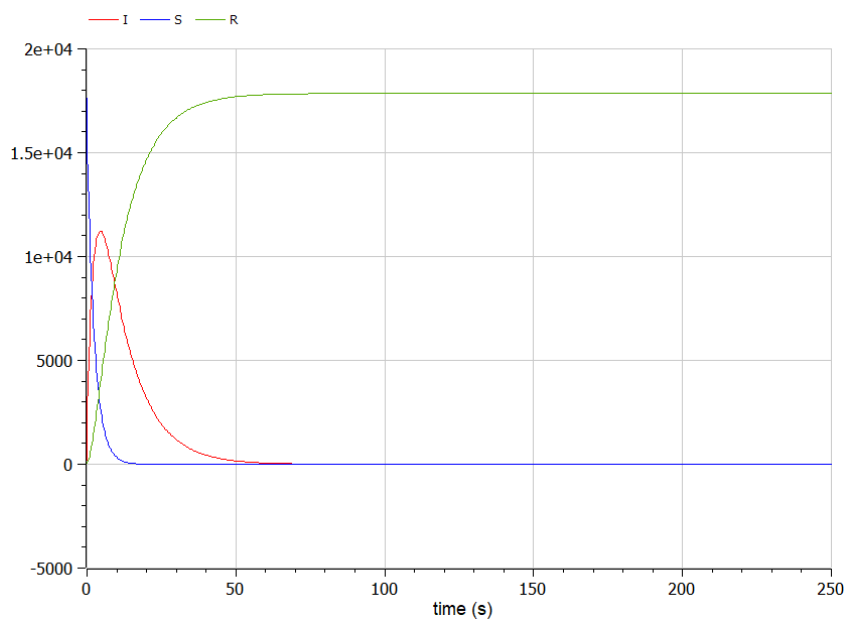
Рис. 0.4: График численности особей трёх групп S, I, R, построенные на OpenModelica, для случая, когда больные могут заражать особей группы S
