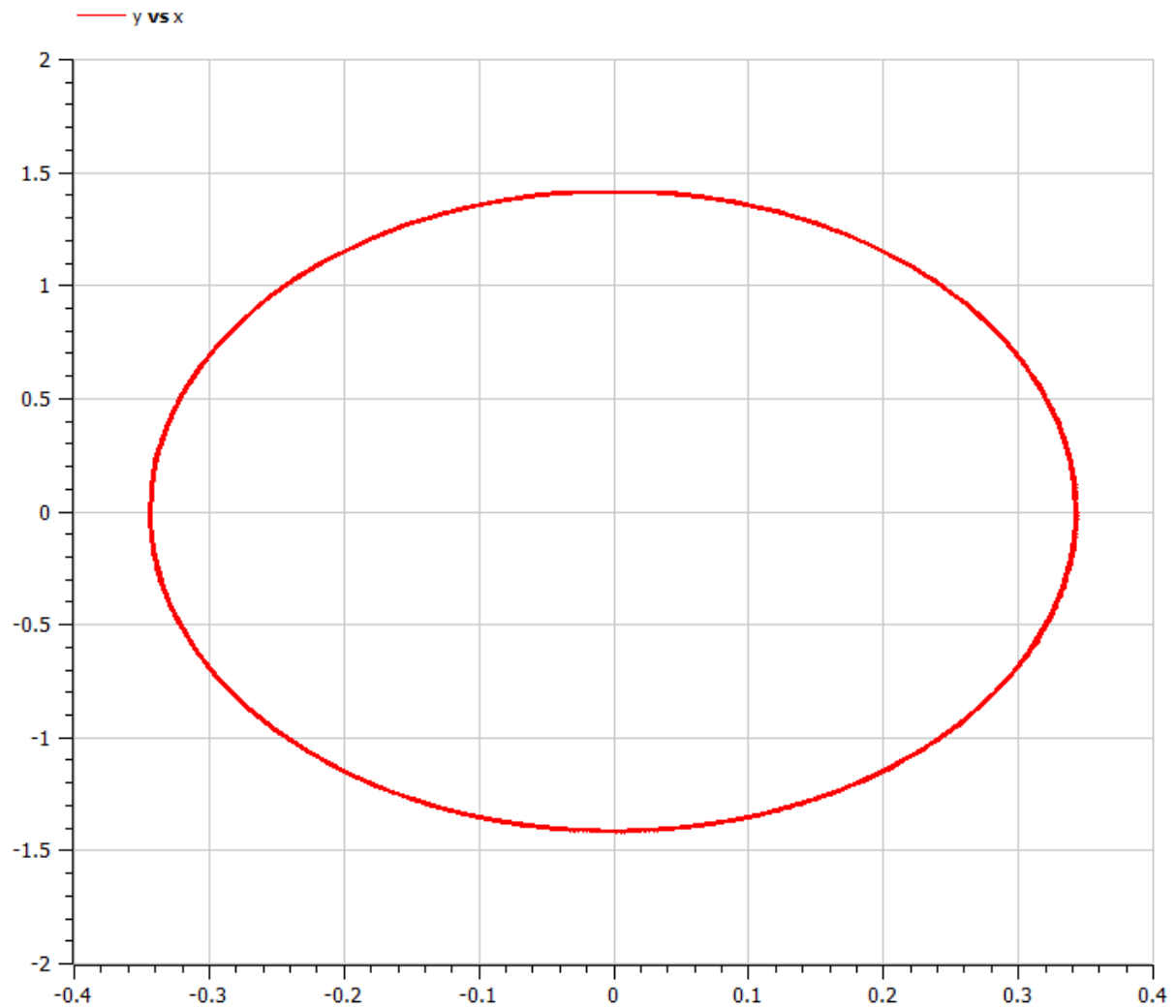
Рис. 0.8: “Фазовый портрет для колебания гармонического осциллятора без затуханий и без действий внешней силы на языке Open Modelica”
