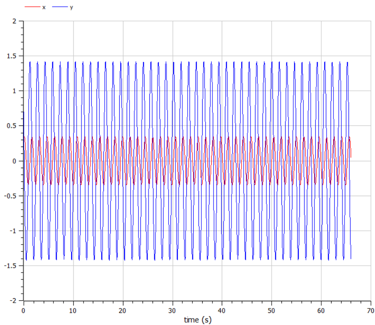
Рис. 0.7: “Решение уравнения для колебания гармонического осциллятора без затуханий и без действий внешней силы на языке Open Modelica”
