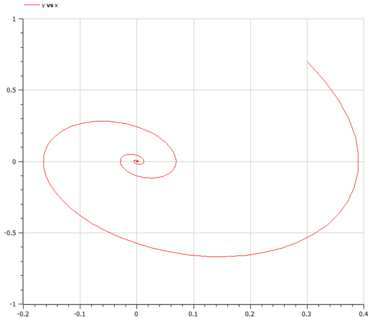
Рис. 0.10: “Фазовый портрет для колебания гармонического осциллятора с затуханием и без действий внешней силы на языке Open Modelica”
