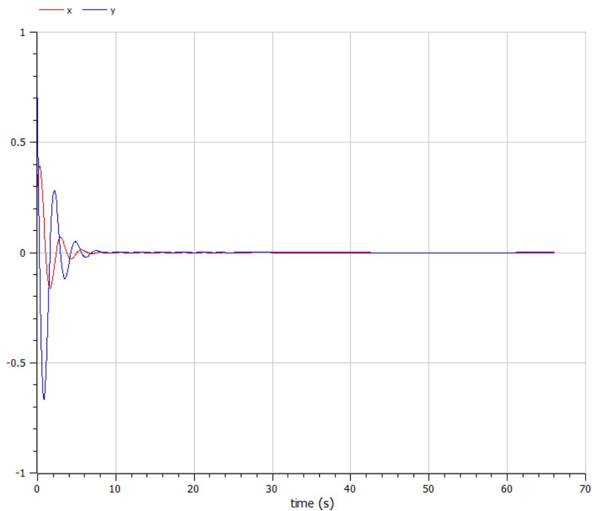
Рис. 0.9: “Решение уравнения для колебания гармонического осциллятора с затуханием и без действий внешней силы на языке Open Modelica”
