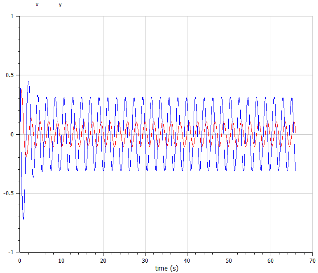
Рис. 0.11: “Решение уравнения для колебания гармонического осциллятора с затуханием и под действием внешней силы на языке Open Modelica”
