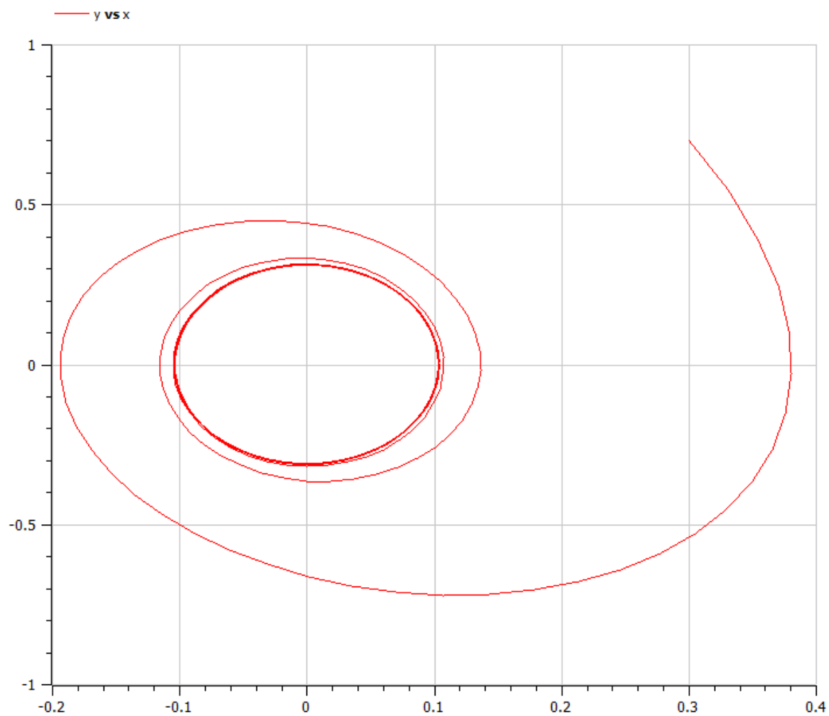
Рис. 0.12: “Фазовый портрет для колебания гармонического осциллятора с затуханием и под действием внешней силы на языке Open Modelica”
