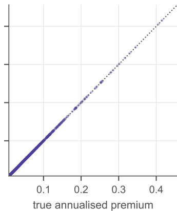
(d) R^2 1.00
