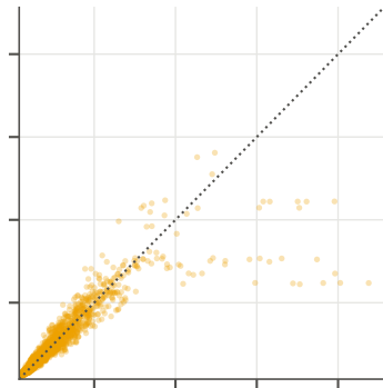
(b) R^2 0.74
