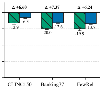
(d) New class orders: BWT feat
