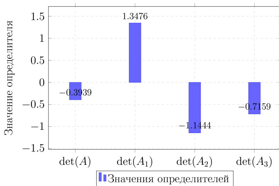
Рис. 2 – Определители матриц для метода Крамера
