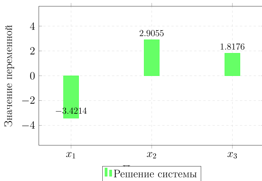
Рис. 3 – Графическое представление решения системы
