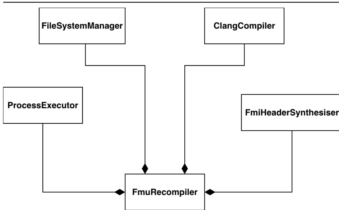
Figura 4.2: Struttura di FmuRecompiler
