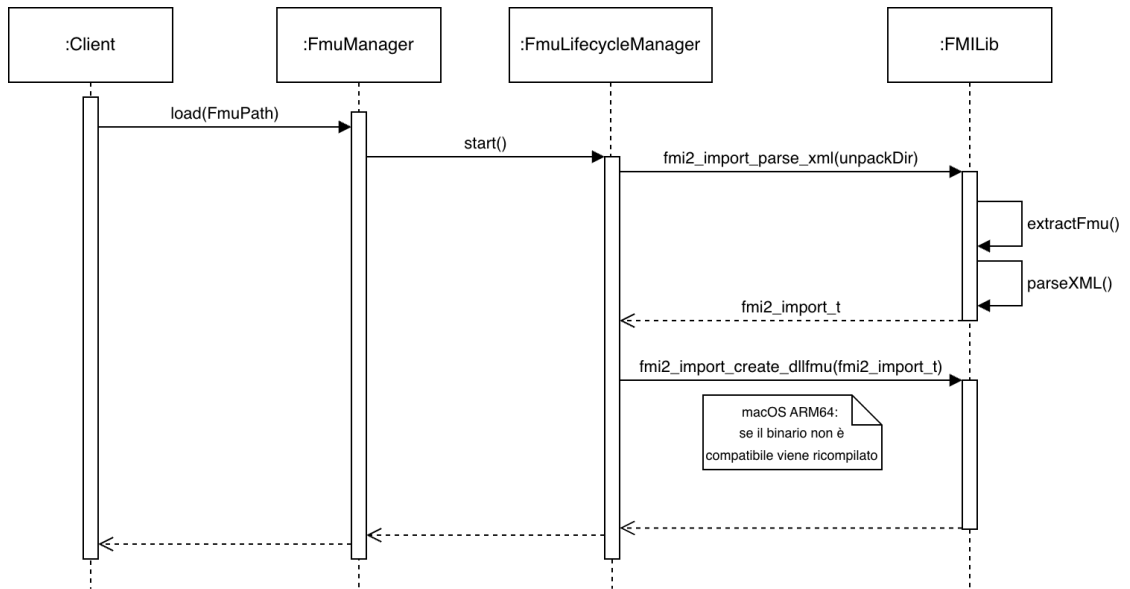
Figura 4.1: Diagramma rappresentante il processo di inizializzazione del ciclo di vita del file FMU.
