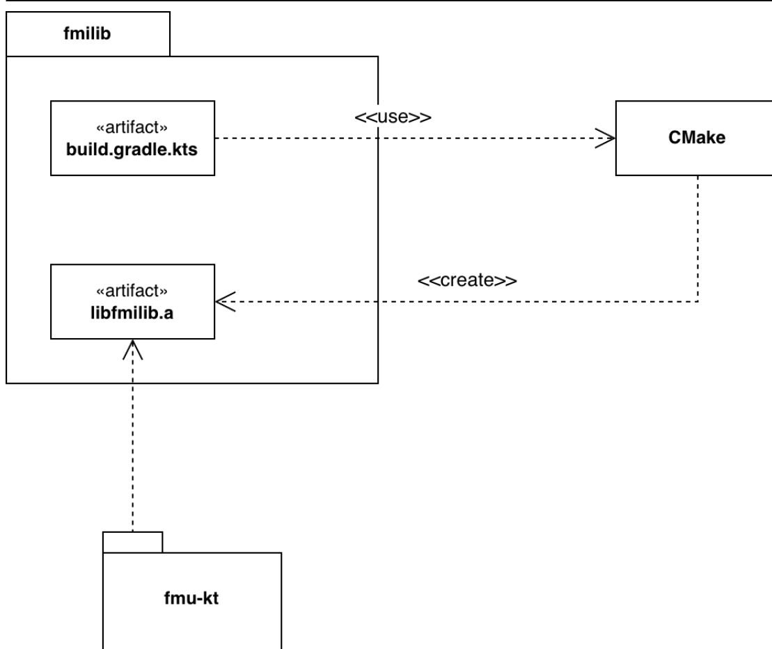
Figura 4.3: Diagramma rappresentante il processo di compilazione della libreria FMILib.
