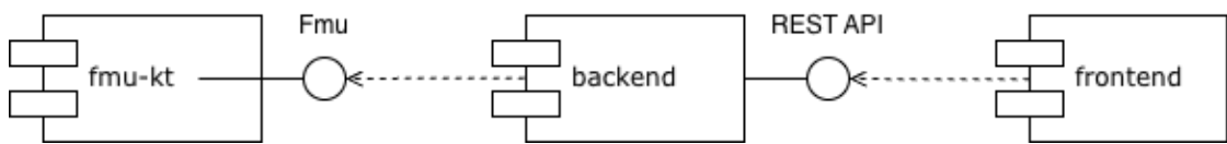
Figure 4.1: Diagramma rappresentante relazione tra i moduli dell'applicativo.
