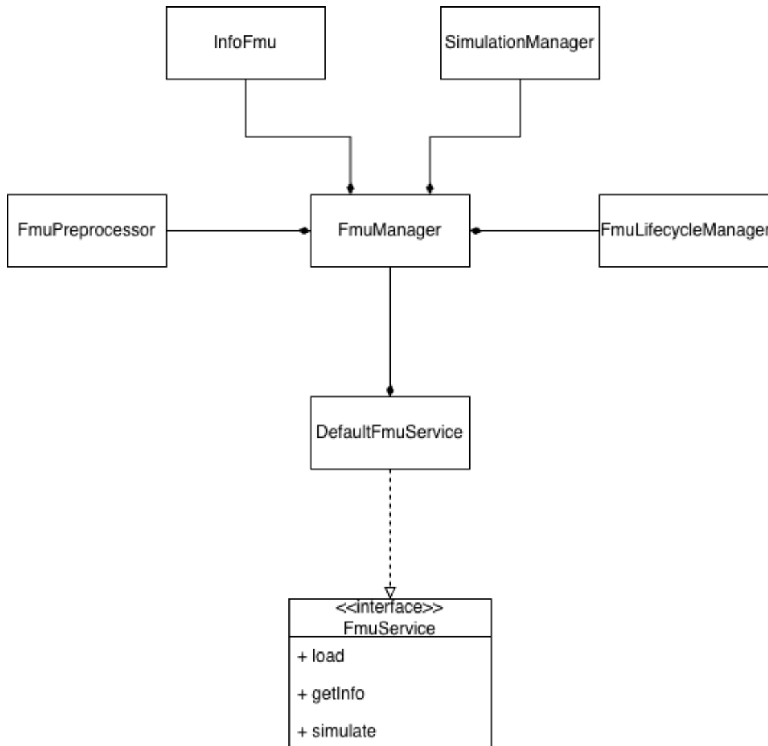
Figure 4.2: Diagramma delle dipendenze di DefaultFmuService
