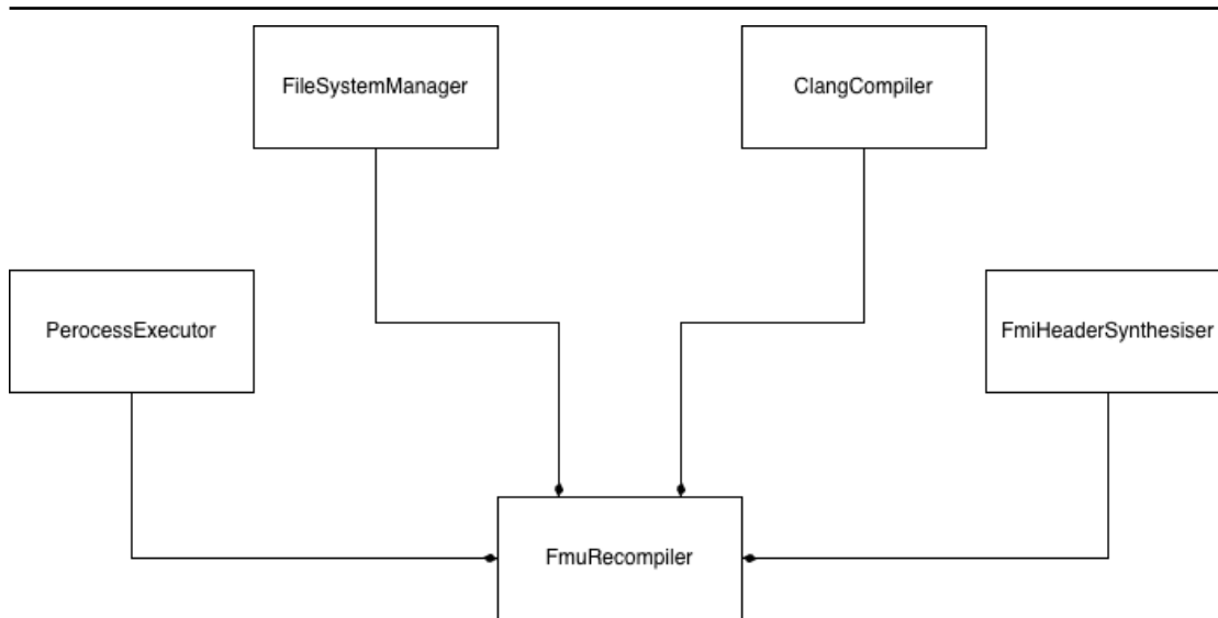
Figure 5.1: Struttura di FmuRecompiler
