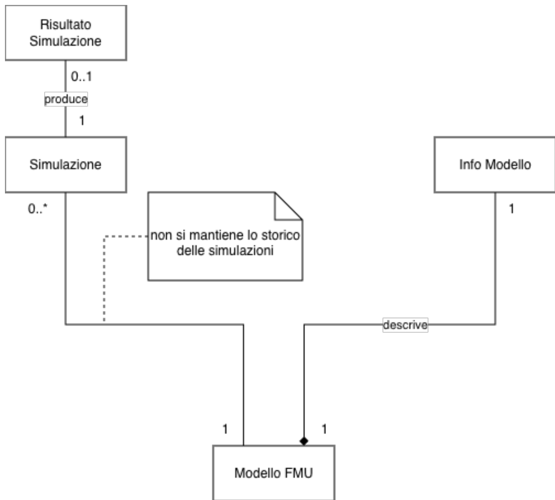
Figure 3.1: Schema rappresentate le entità del modello del dominio.
