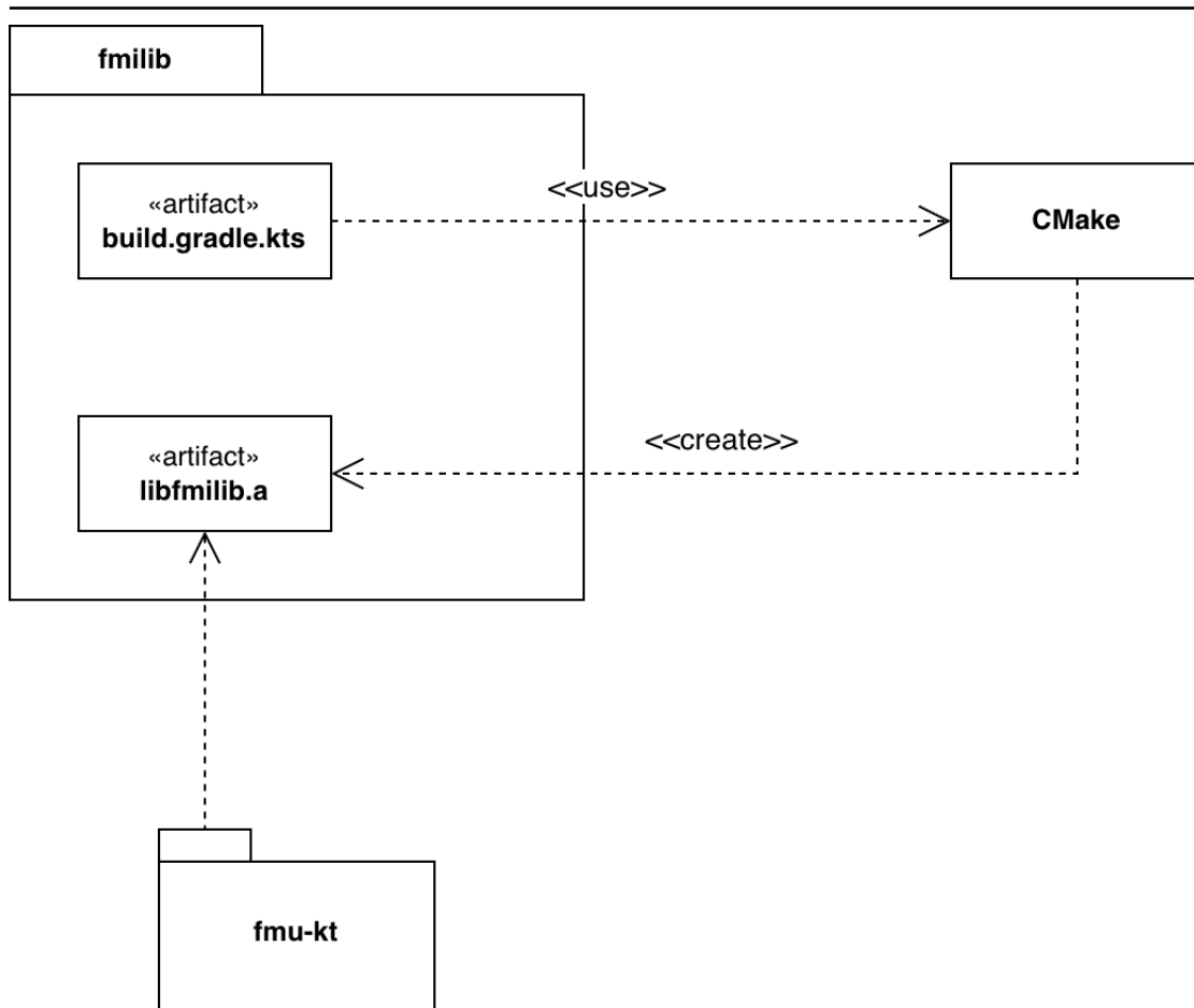
Figure 4.2: Diagramma rappresentante il processo di compilazione della libreria FMILib.
