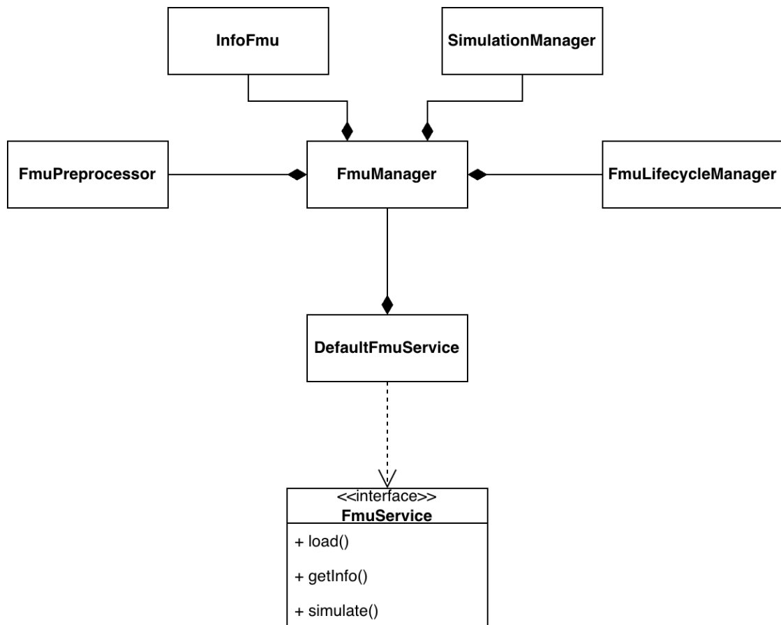
Figure 3.2: Diagramma delle dipendenze di DefaultFmuService
