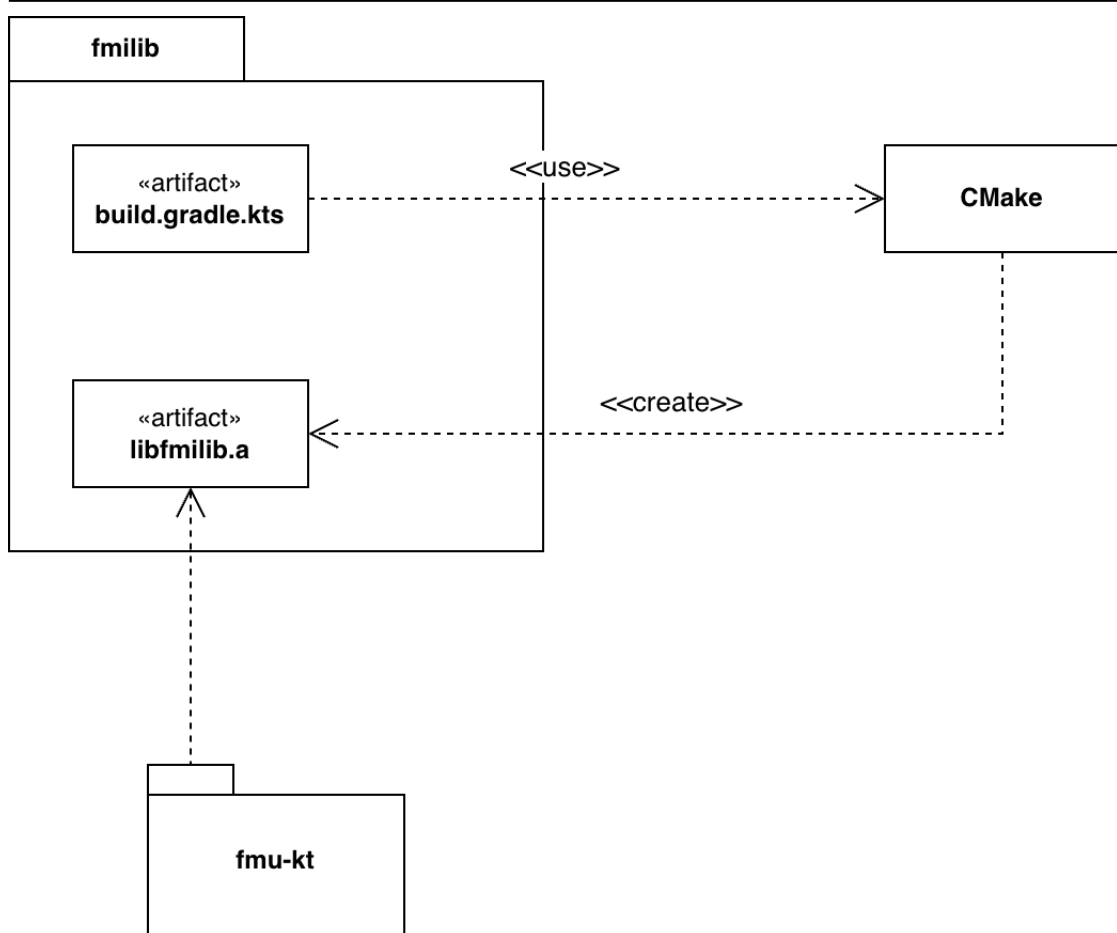
Figure 5.2: Diagramma rappresentante il processo di compilazione della libreria FMILib.
