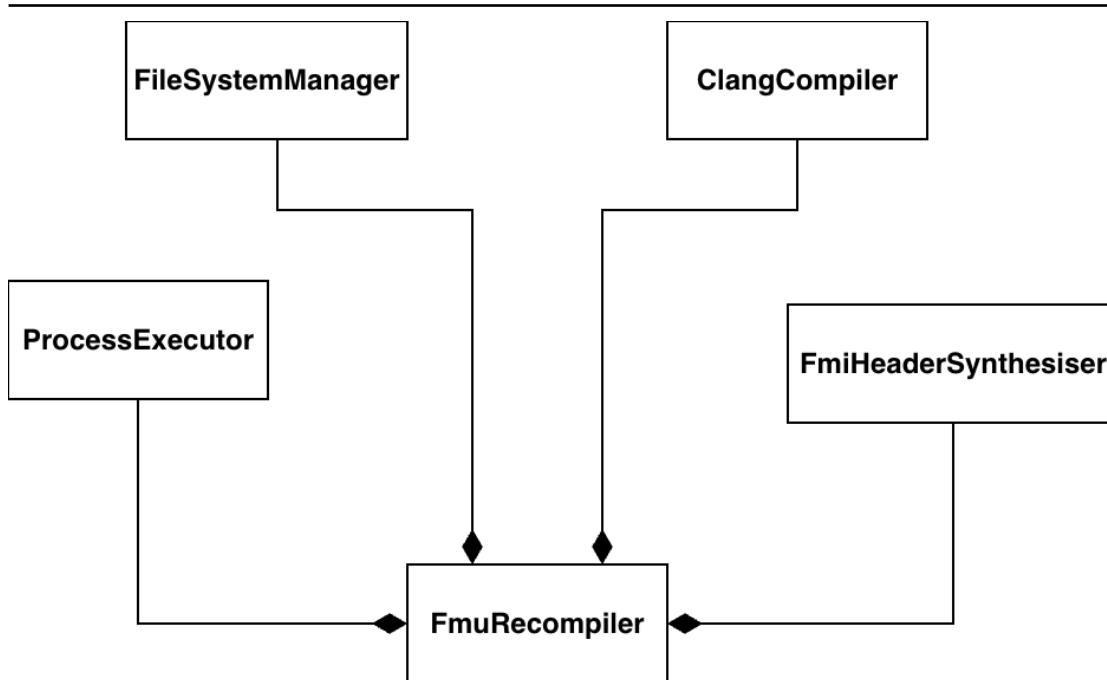
Figure 5.1: Struttura di FmuRecompiler
