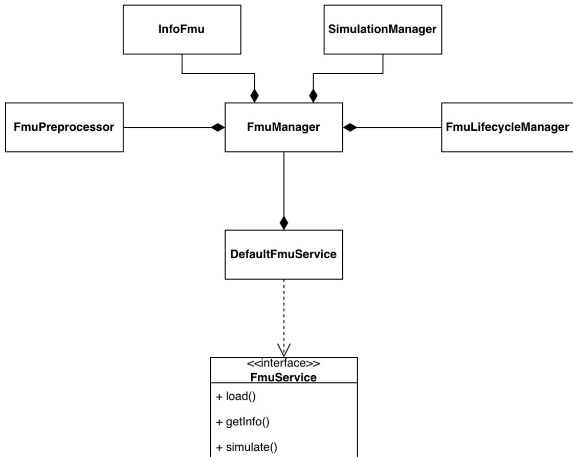
Figure 4.2: Diagramma delle dipendenze di DefaultFmuService
