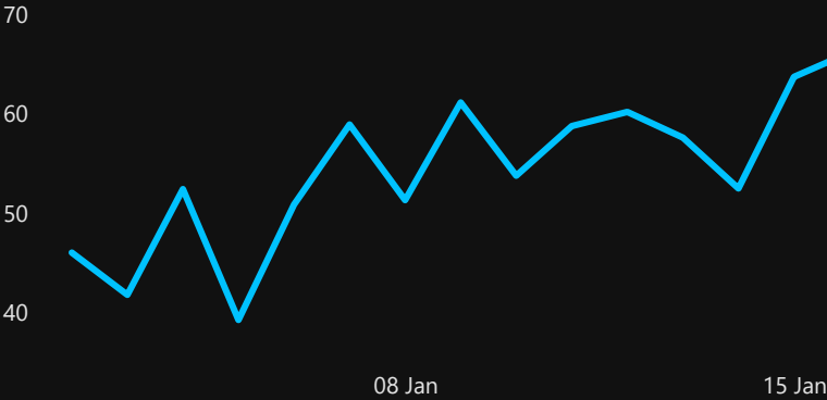
RSI Trend
