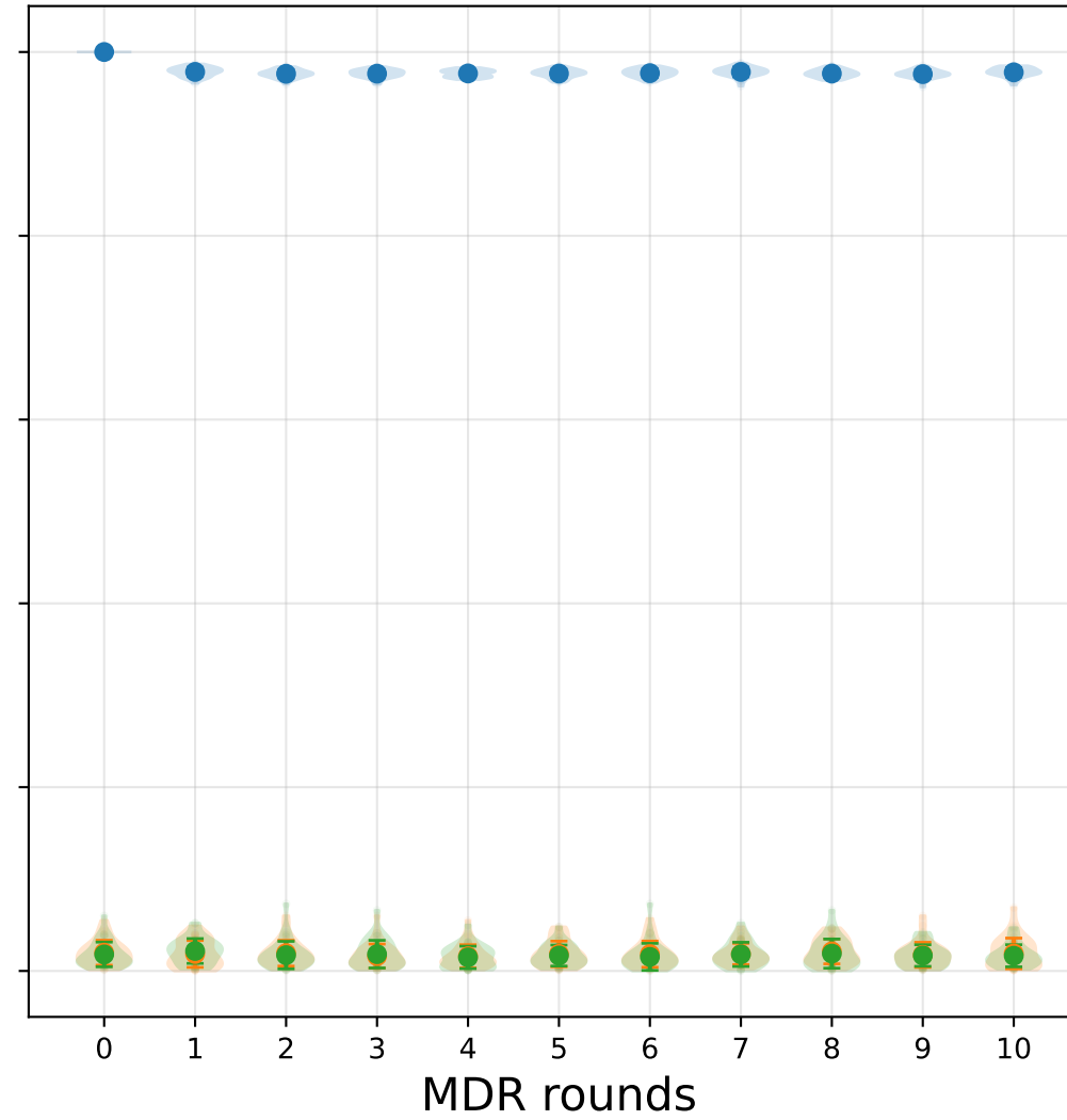
Pure Z Noise
