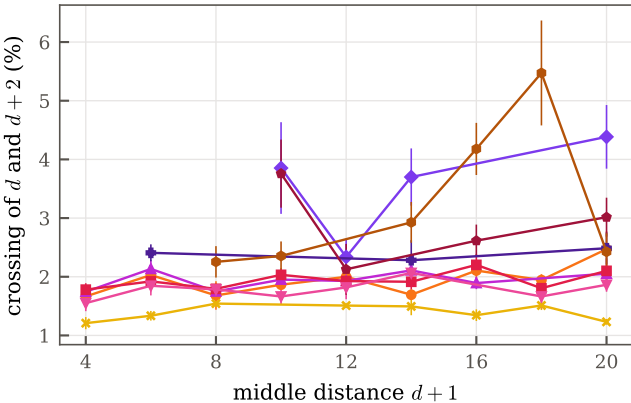
r = 1 , Pure Z
