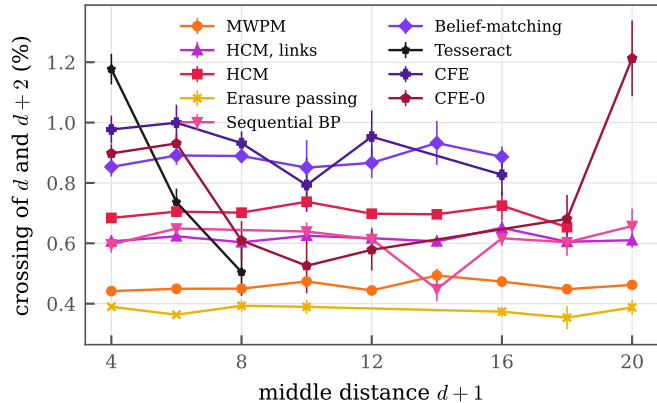
r = d , Pure Z
