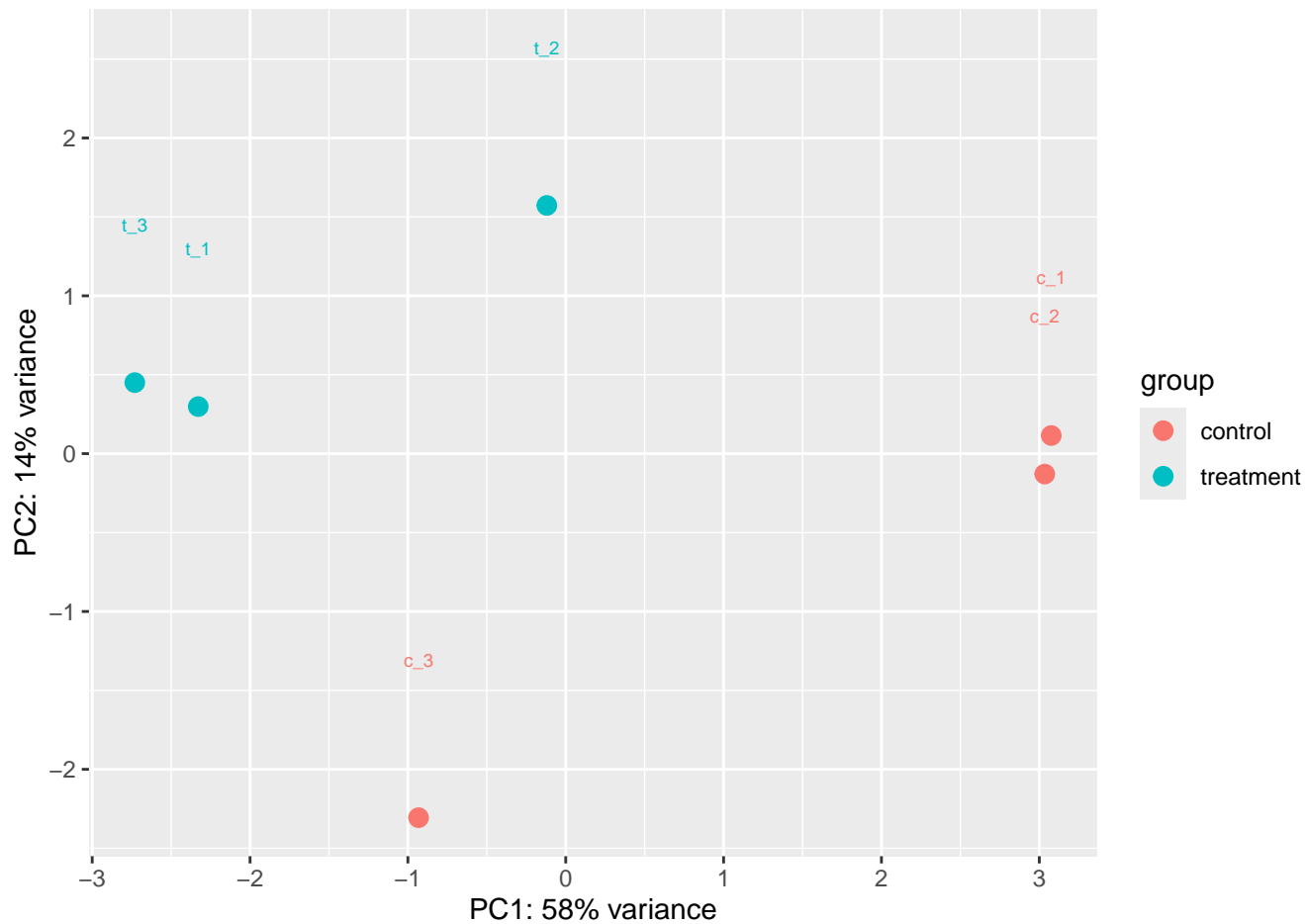
PCA plot
