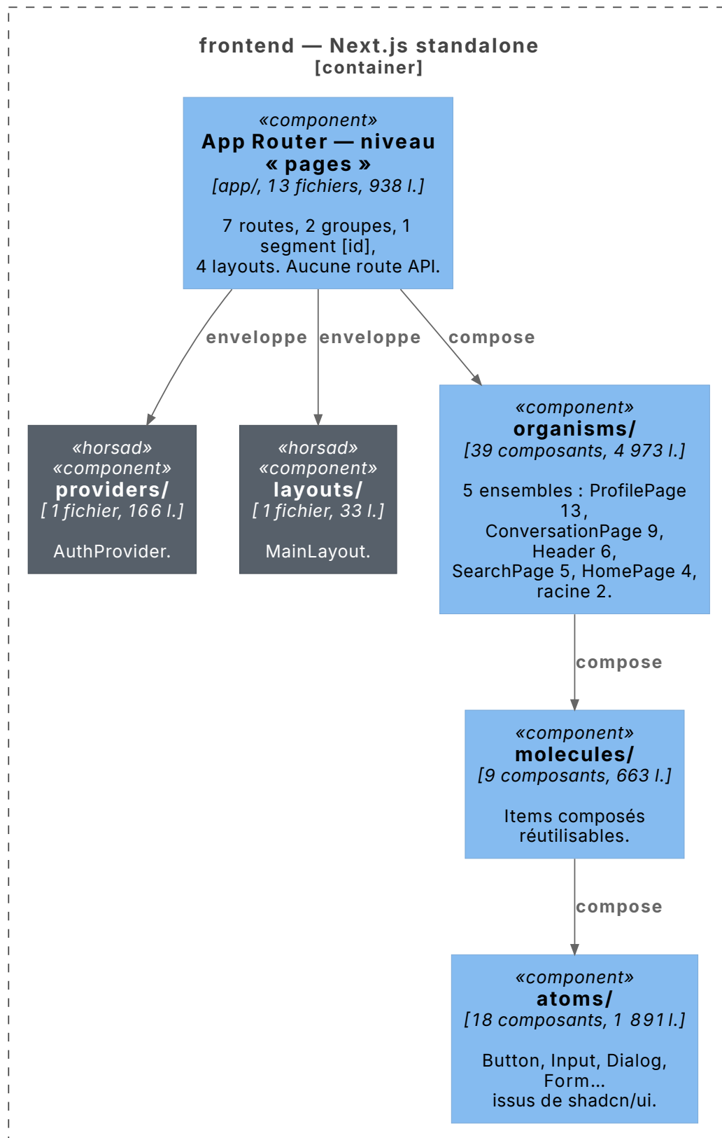
Fig. 13. – C4 niveau 3, frontend vue 1/2 — composition de l'interface. Chaque niveau porte son nombre de composants, barils index.ts exclus, selon la même convention de comptage que le lexique 15. En gris, les deux répertoires de components/ qui ne sont pas des niveaux Atomic Design. Couture : l'App Router et les organismes sont repris en Fig. 14.
