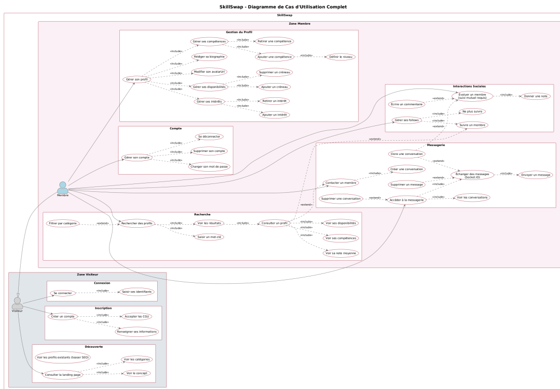
Fig. 11. – Diagramme de cas d'utilisation de SkillSwap. Deux acteurs : le visiteur non-authentifié et le membre authentifié. Les cas d'utilisation grisés sont hors-scope MVP et reportés à la V2.
