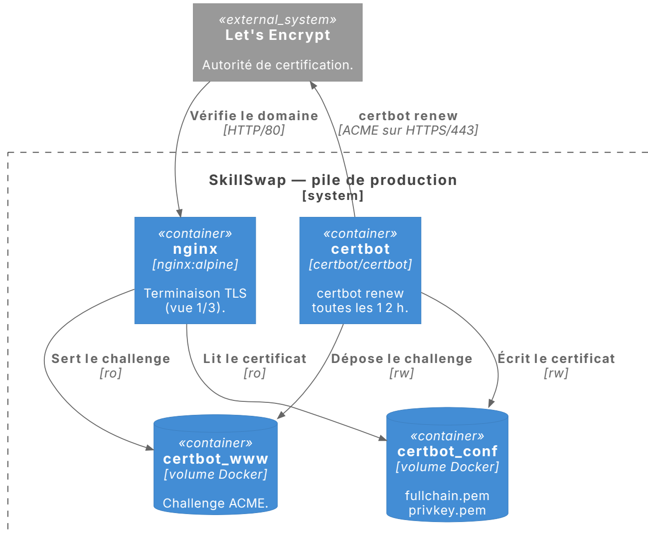
Fig. 4. – C4 niveau 2, vue 3/3 — chaîne de renouvellement TLS . Couture avec Fig. 2 : le conteneur nginx , qui assure la terminaison TLS. Les deux volumes certbot sont montés deux fois — en écriture côté certbot, en lecture seule côté nginx.
