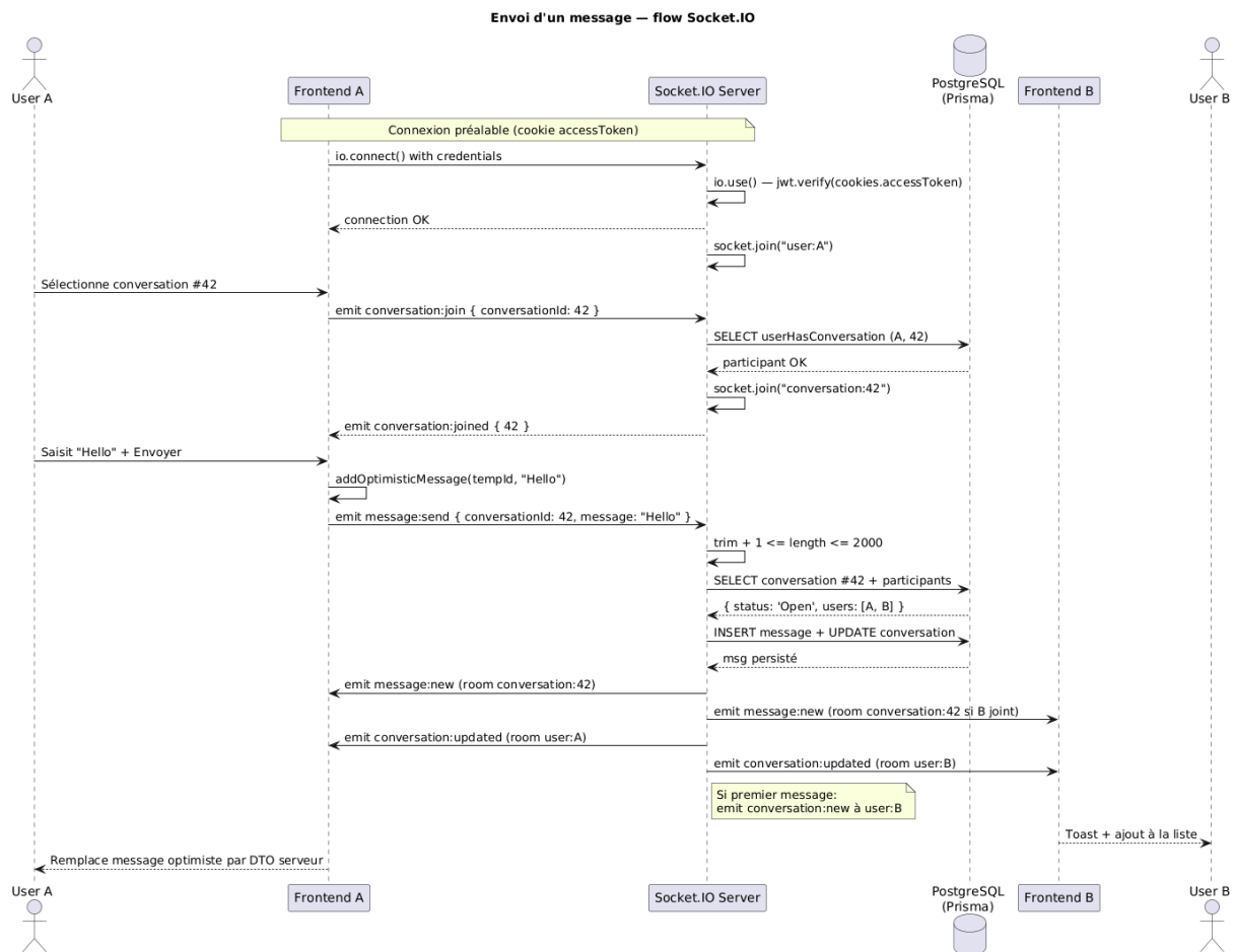
Fig. 18. – Diagramme de séquence de l'envoi d'un message — flux complet : authentification socket, optimistic UI, validation serveur, persistance Prisma, diffusion multi-rooms.
