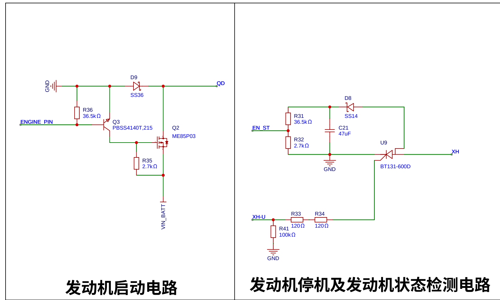
发动机启动电路
