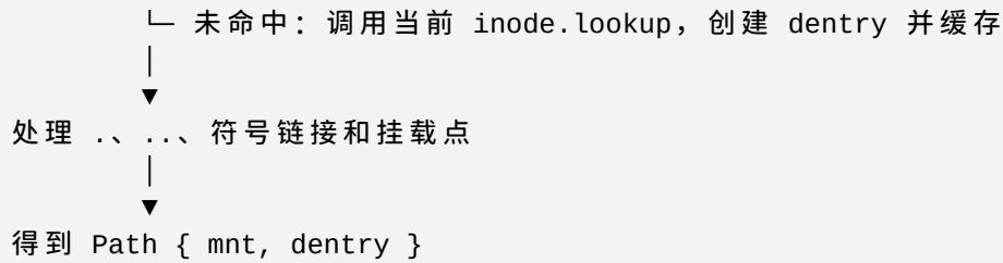
图 5-2 namei 路径解析流程
