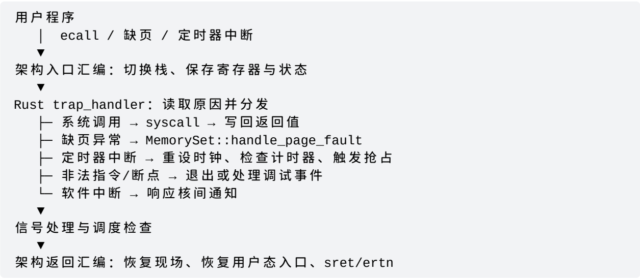
图 3-1 用户态 trap 的入口、分发与返回路径
