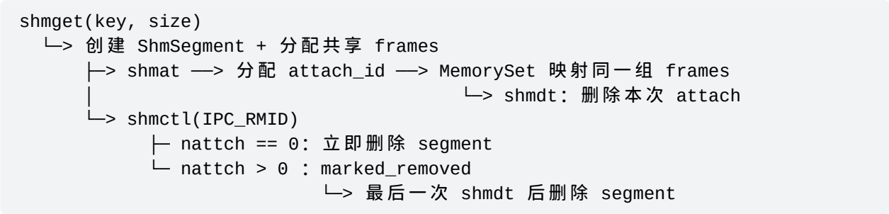
图 6-3 System V 共享内存生命周期
