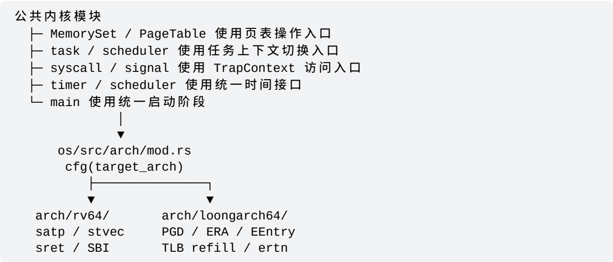
图 9-1 RespOS 双架构适配结构
