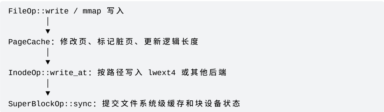
图 5-3 文件写入与持久化写回链路
