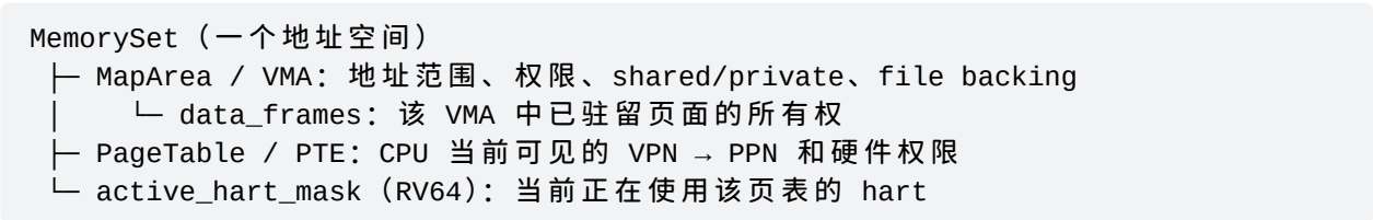
图 4-1 MemorySet、VMA、PTE 与驻留页的层次关系
