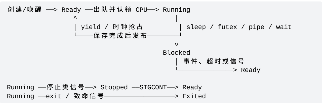
图 2-2 任务状态转换
