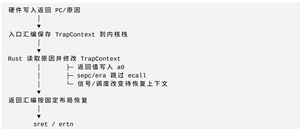
图 3-2 TrapContext 在一次 trap 中的生命周期
