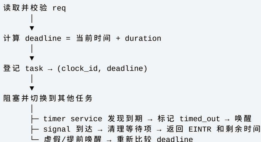
图 7-2 nanosleep 的登记、唤醒与返回流程
