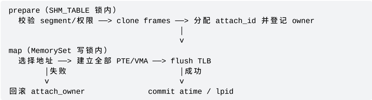
图 6-4 shmat 的 prepare/commit 协议
