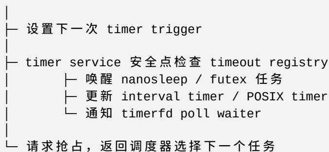
图 7-1 时钟中断到超时处理的调用链
