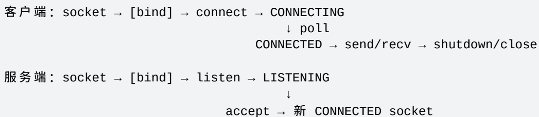
图 8-3 TCP 客户端与服务端生命周期
