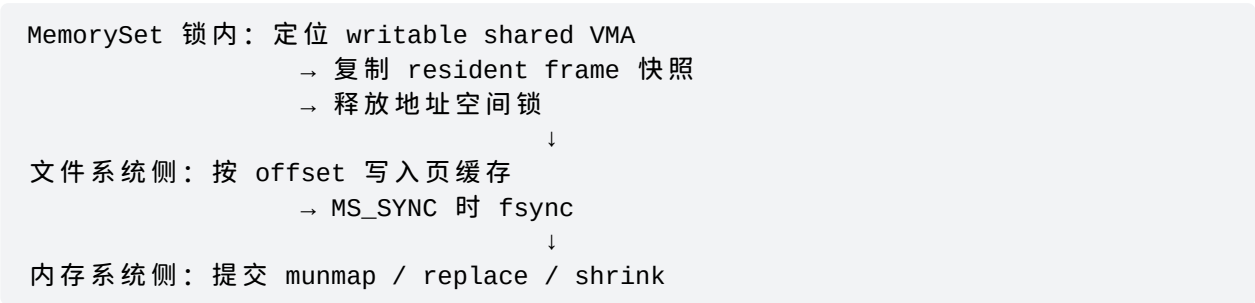
图 4-4 共享文件页的锁外写回协议
