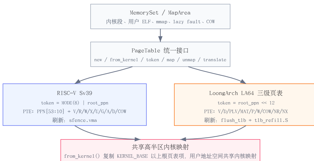
图 24 MemorySet 与架构页表后端
