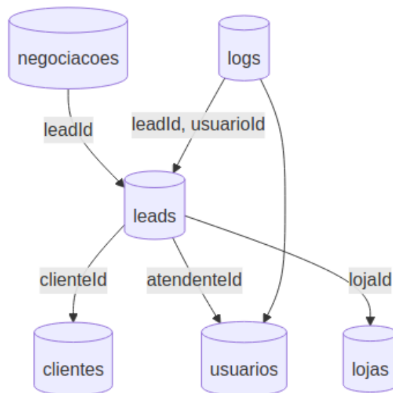
Figura 2 – Visão geral das coleções e referências.
