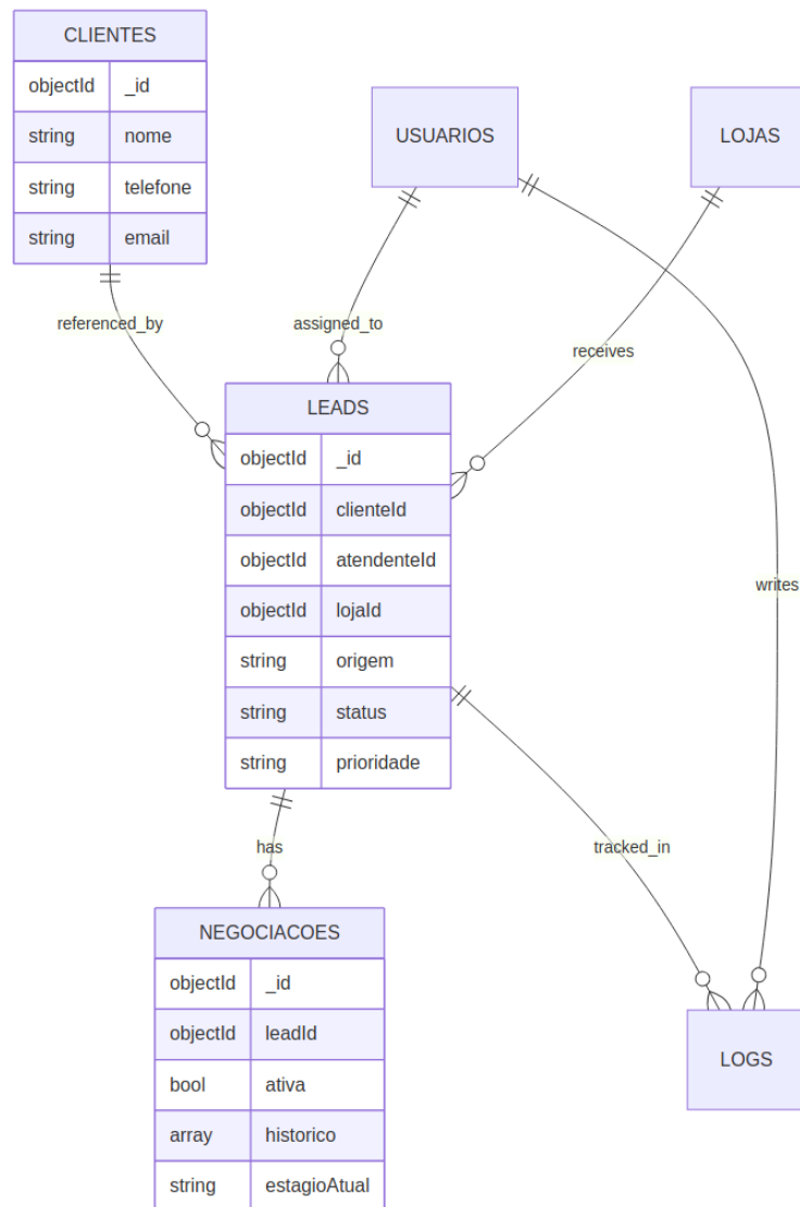
Figura 3 – Entidades, atributos e cardinalidades.
