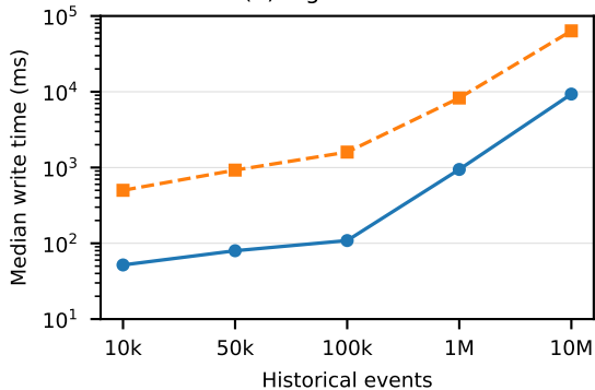
(d) Ingestion time
