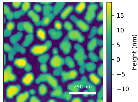
measured AFM Rq=9.87 nm, FSMI=8.57 nm
