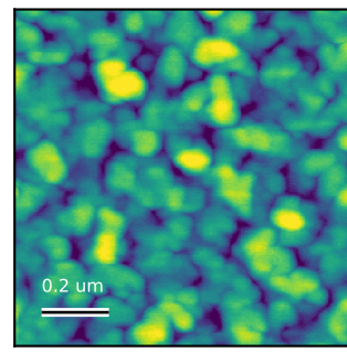
AFM Rq = 2.019 nm Scan: 1 x 1 um
