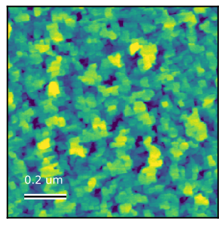
AFM Rq = 1.274 nm Scan: 1 x 1 um
