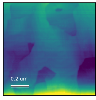
AFM Rq = 2.127 nm Scan: 1 x 1 um
