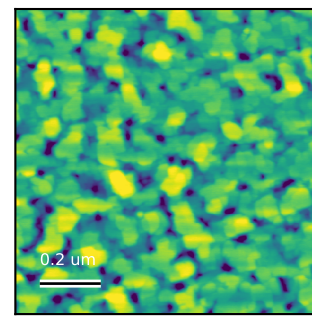
AFM Rq = 3.177 nm Scan: 1 x 1 um
