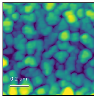
AFM Rq = 3.095 nm Scan: 1 x 1 um
