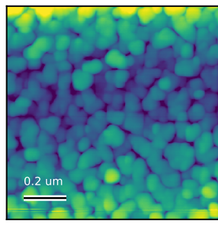
AFM Rq = 2.473 nm Scan: 1 x 1 um
