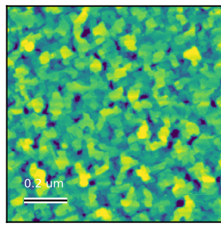
AFM Rq = 1.832 nm Scan: 1 x 1 um
