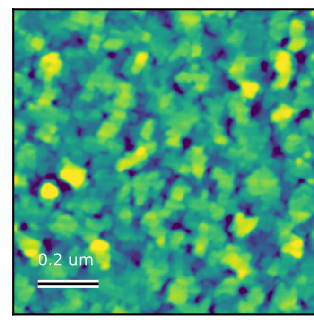
AFM Rq = 1.638 nm Scan: 1 x 1 um
