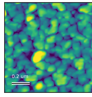
AFM Rq = 1.864 nm Scan: 1 x 1 um
