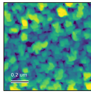
AFM Rq = 2.561 nm Scan: 1 x 1 um
