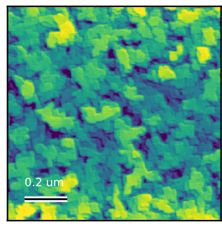
AFM Rq = 3.047 nm Scan: 1 x 1 um
