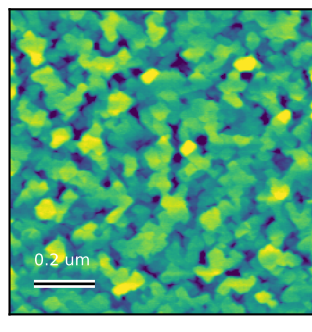
AFM Rq = 1.470 nm Scan: 1 x 1 um
