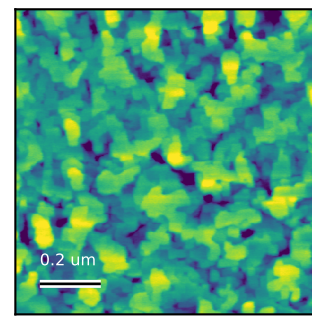
AFM Rq = 1.517 nm Scan: 1 x 1 um
