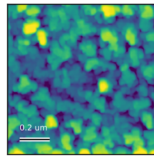
AFM Rq = 2.529 nm Scan: 1 x 1 um
