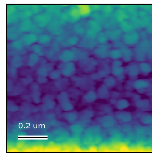
AFM Rq = 3.181 nm Scan: 1 x 1 um
