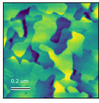
AFM Rq = 1.649 nm Scan: 1 x 1 um
