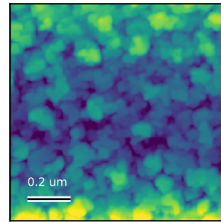
AFM Rq = 3.227 nm Scan: 1 x 1 um
