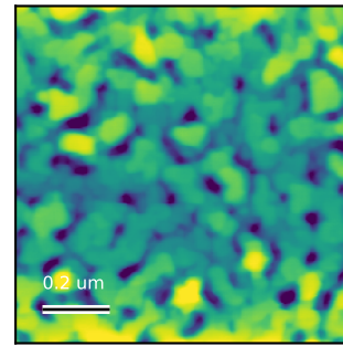
AFM Rq = 5.159 nm Scan: 1 x 1 um
