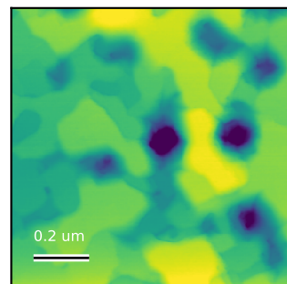
AFM Rq = 10.290 nm Scan: 1 x 1 um
