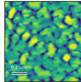
AFM Rq = 4.127 nm Scan: 1 x 1 um
