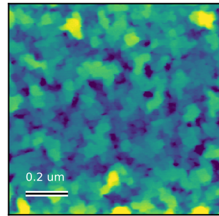
AFM Rq = 3.225 nm Scan: 1 x 1 um
