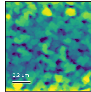
AFM Rq = 5.337 nm Scan: 1 x 1 um
