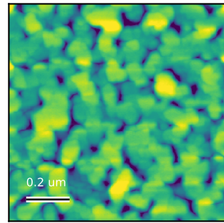
AFM Rq = 4.693 nm Scan: 1 x 1 um
