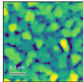
AFM Rq = 6.073 nm Scan: 1 x 1 um
