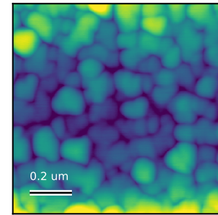
AFM Rq = 4.685 nm Scan: 1 x 1 um
