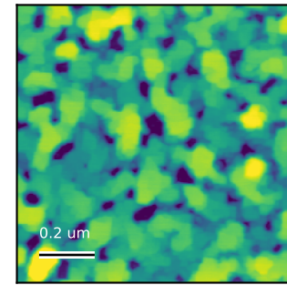
AFM Rq = 6.004 nm Scan: 1 x 1 um
