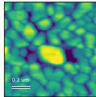
AFM Rq = 7.372 nm Scan: 1.02 x 1.02 um
