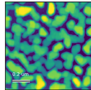
AFM Rq = 9.867 nm Scan: 1 x 1 um
