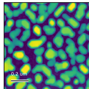
AFM Rq = 10.321 nm Scan: 1 x 1 um
