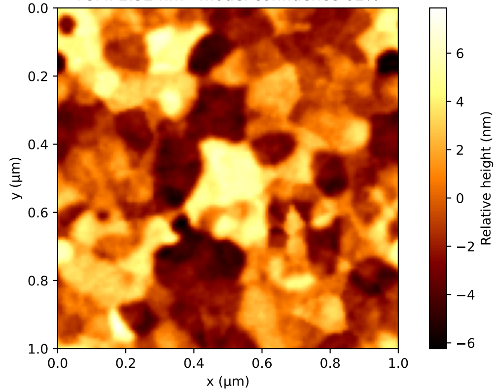
Generated AFM · Rq 2.69 nm FSMI 2.32 nm · model confidence 62%
