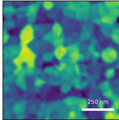
generated AFM Rq=1.42 nm, FSMI=1.08 nm, C=52/100
