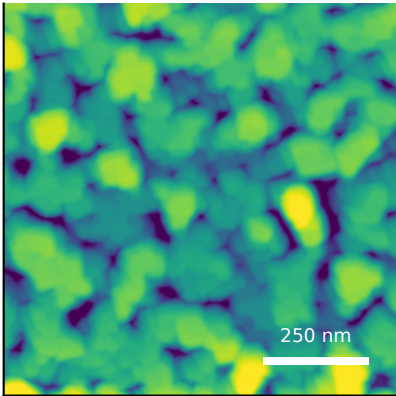
measured AFM Rq=9.87 nm, FSMI=8.57 nm
