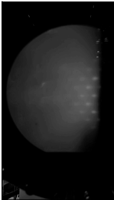
6033 RHEED key frame
