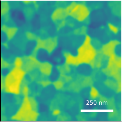
generated AFM Rq=3.44 nm, FSMI=2.45 nm, C=93/100
