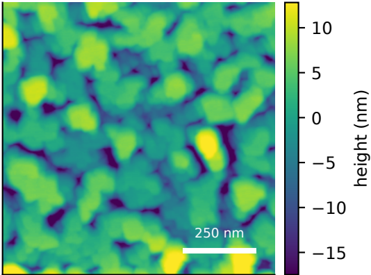
measured AFM Rq=9.87 nm, FSMI=8.57 nm
