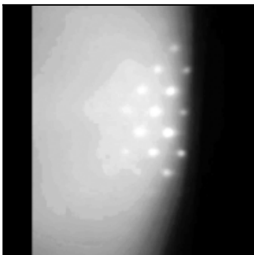
auto RHEED | Cq=72
