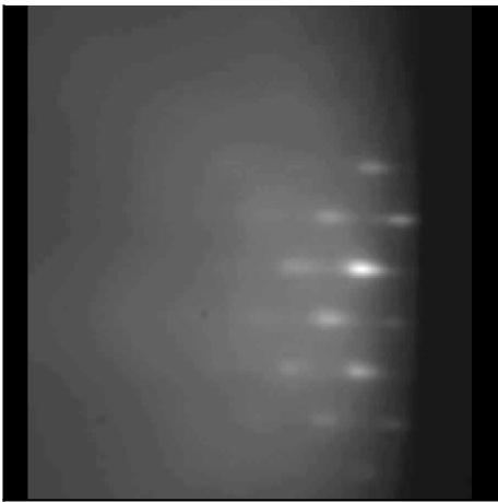
N6358 RHEED key frame
