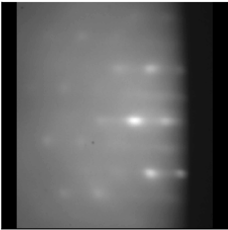
N6382 RHEED key frame
