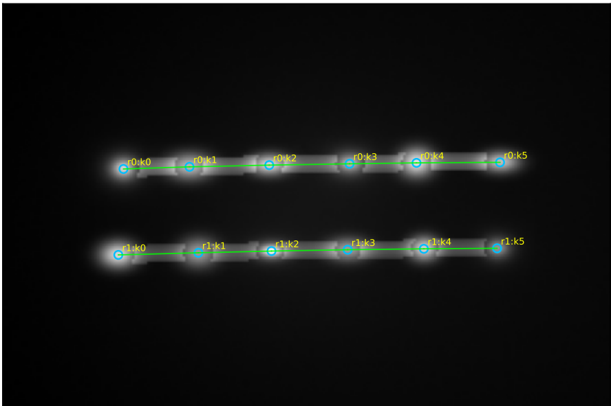
challenge_valid_near_missing_site
