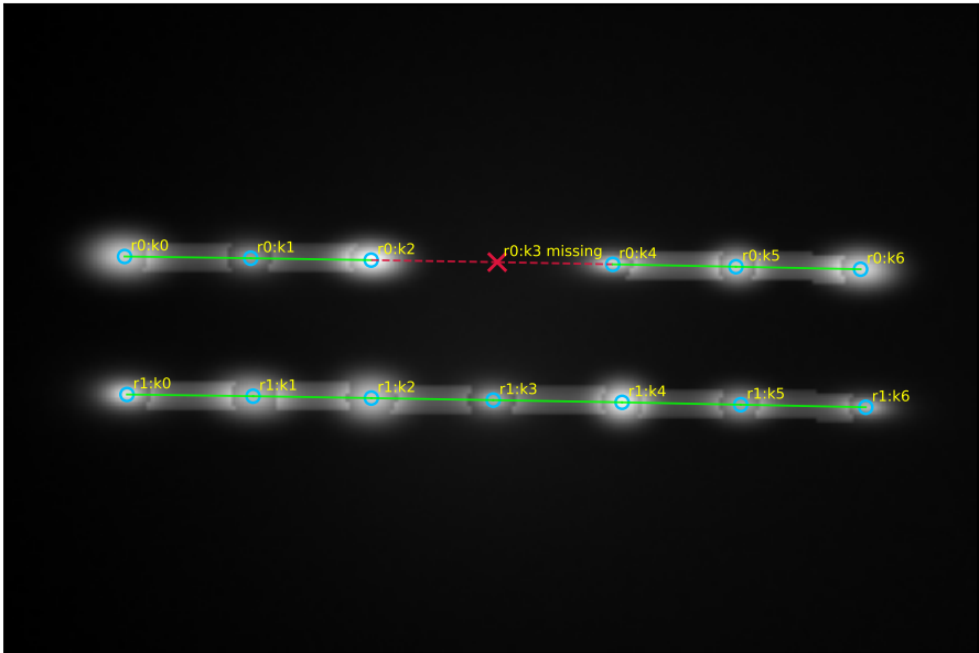
challenge_duplicate_local_maximum
