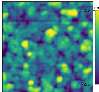
N6358 GT 5 Rq = 1.12 nm
