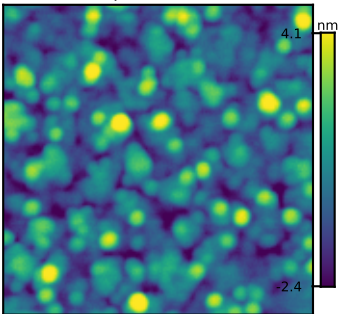
N6382 GT 1 Rq = 1.37 nm
