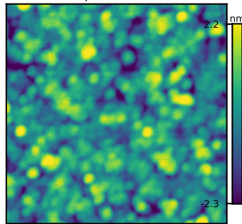
N6342 GT 3 Rq = 0.92 nm
