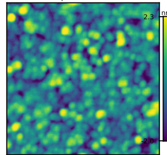
N6342 GT 4 Rq = 0.88 nm
