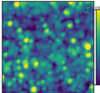
N6382 GT 5 Rq = 1.35 nm
