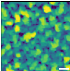
6029 true
