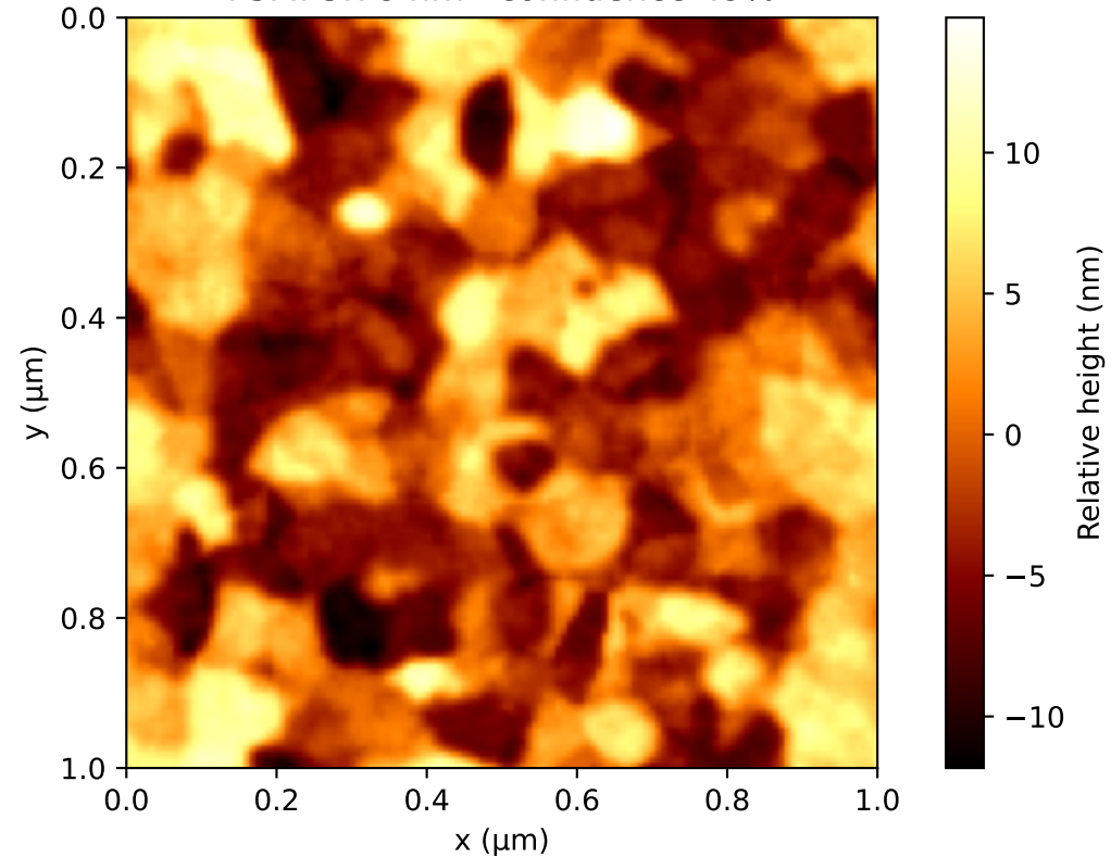
Generated AFM · Rq 5.21 nm FSMI 3.78 nm · confidence 49%
